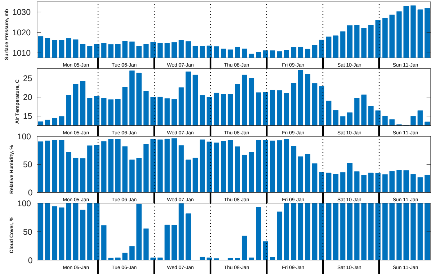
Met Forecast for Brooks McCall from 05-Jan-2026 00:00:00 to 12-Jan-2026 00:00:00
