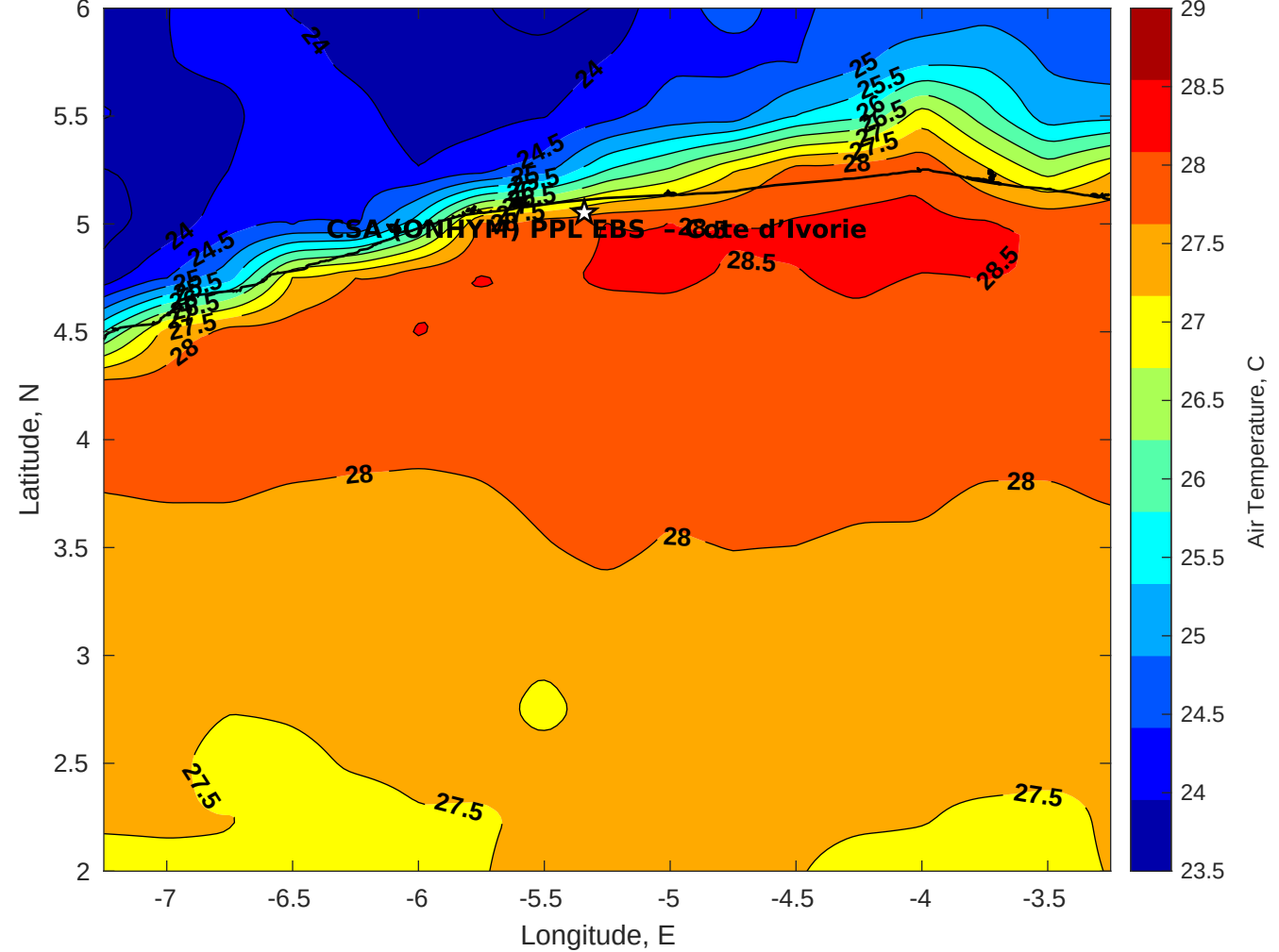
Air Temperature (C) for CSA (ONHYM) PPL EBS - Cote d'Ivoire at 05-Jan-2026
