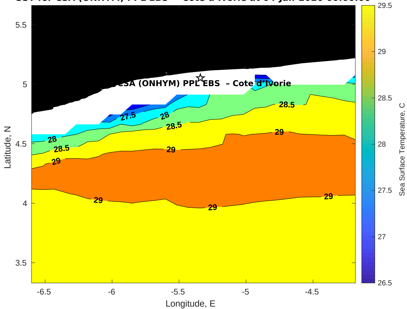
SST for CSA (ONHYM) PPL EBS - Cote d'Ivoire at 04-Jan-2026 00:00:00
