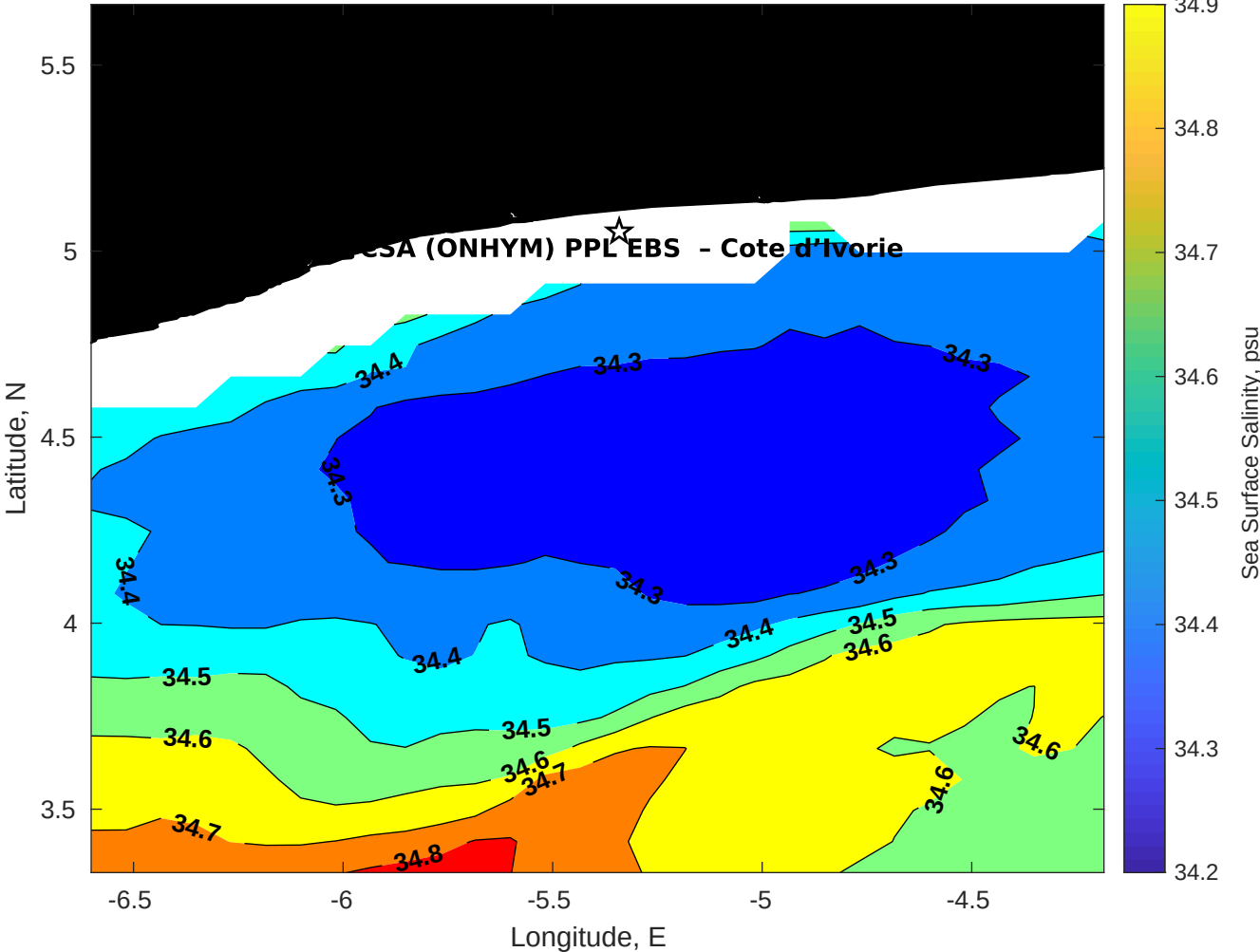
Surface Salinity for CSA (ONHYM) PPL EBS - Cote d'Ivoire at 04-Jan-2026 00:00:00
