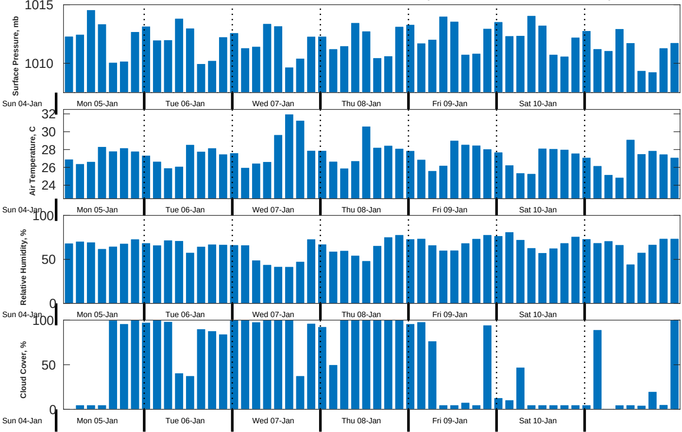
Met Forecast for CSA (ONHYM) PPL EBS - Guinea from 05-Jan-2026 00:00:00 to 12-Jan-2026 00:00:00
