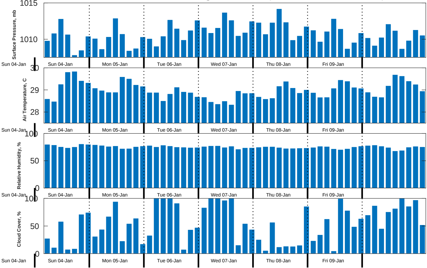
Met Forecast for CSA (ONHYM) PPL EBS - Nigeria from 05-Jan-2026 00:00:00 to 12-Jan-2026 00:00:00
