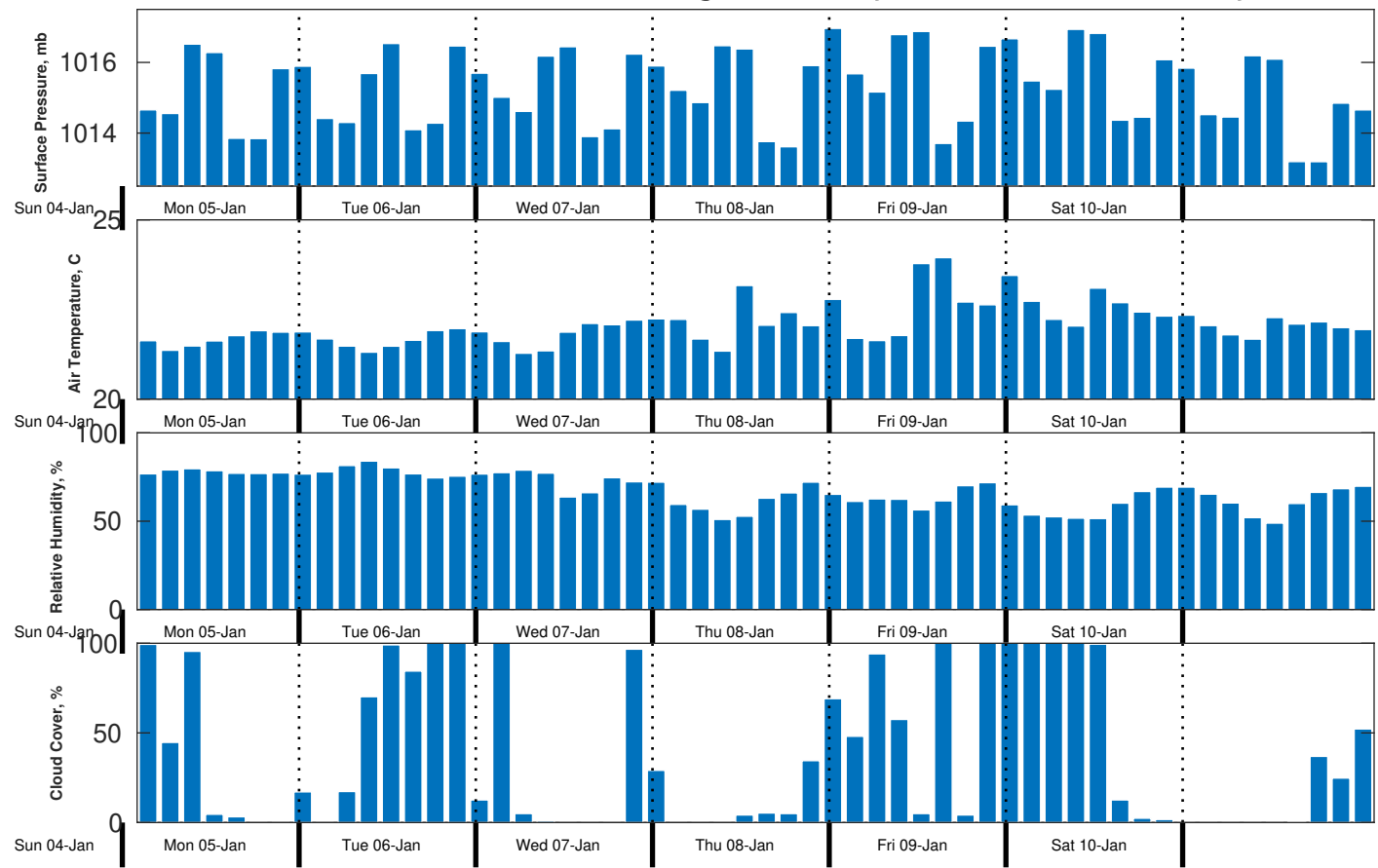
Met Forecast for CSA (ONHYM) PPL EBS - Senegal from 05-Jan-2026 00:00:00 to 12-Jan-2026 00:00:00
