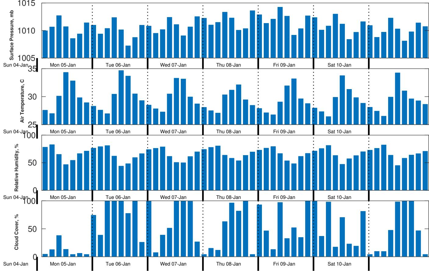
Met Forecast for Proteus from 05-Jan-2026 00:00:00 to 12-Jan-2026 00:00:00
