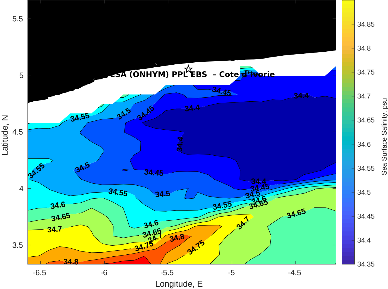
Surface Salinity for CSA (ONHYM) PPL EBS - Cote d'Ivoire at 05-Jan-2026 00:00:00
