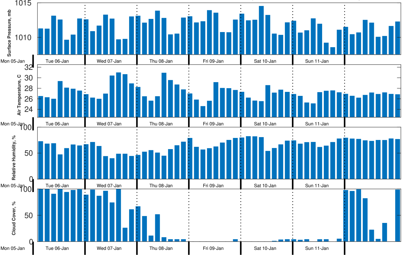
Met Forecast for CSA (ONHYM) PPL EBS - Guinea from 06-Jan-2026 00:00:00 to 13-Jan-2026 00:00:00
