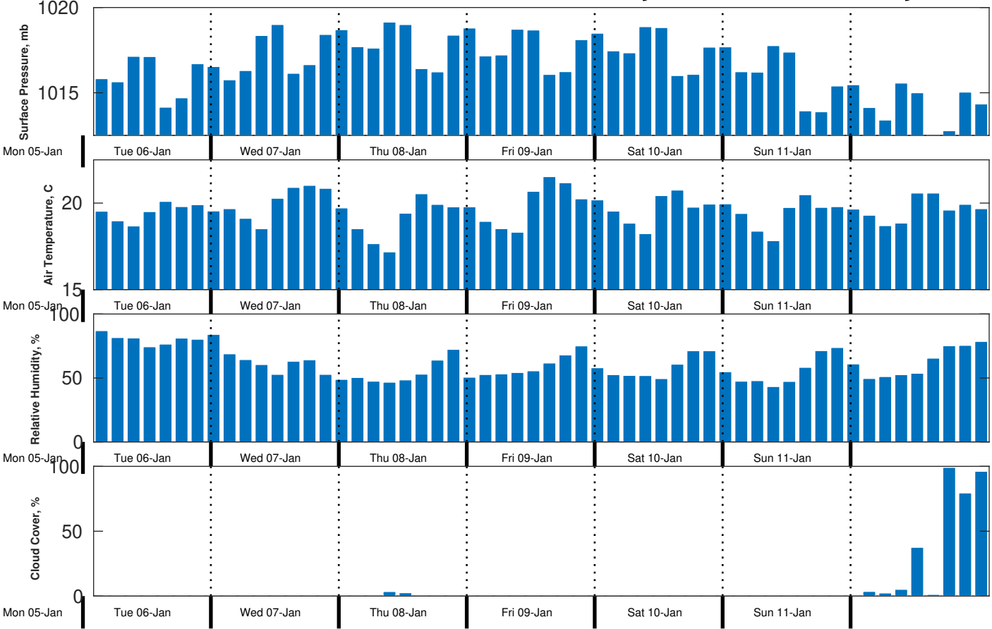
Met Forecast for CSA (ONHYM) PPL EBS - Mauritania from 06-Jan-2026 00:00:00 to 13-Jan-2026 00:00:00
