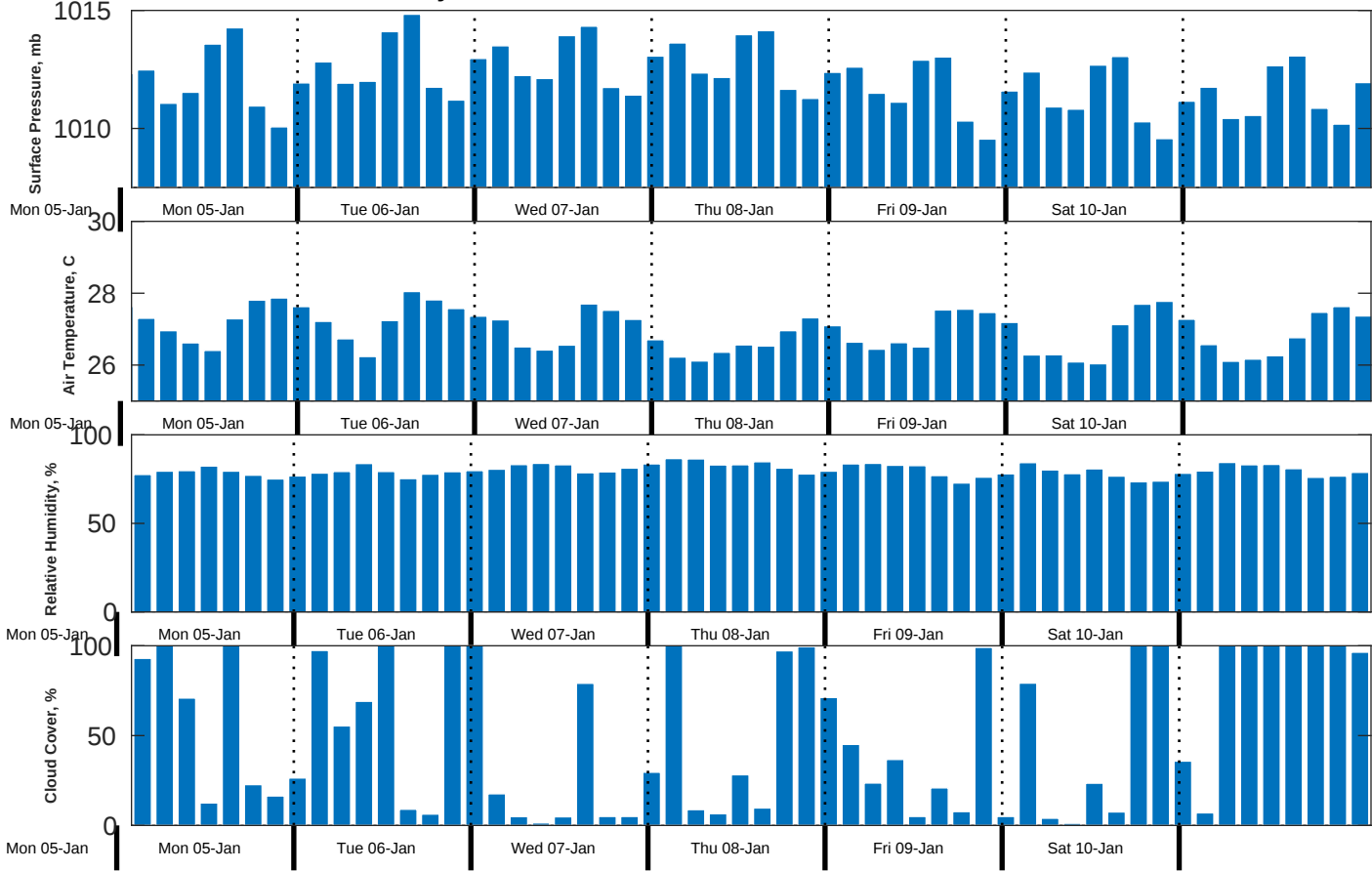
Met Forecast for Gyre from 05-Jan-2026 20:00:00 to 12-Jan-2026 20:00:00
