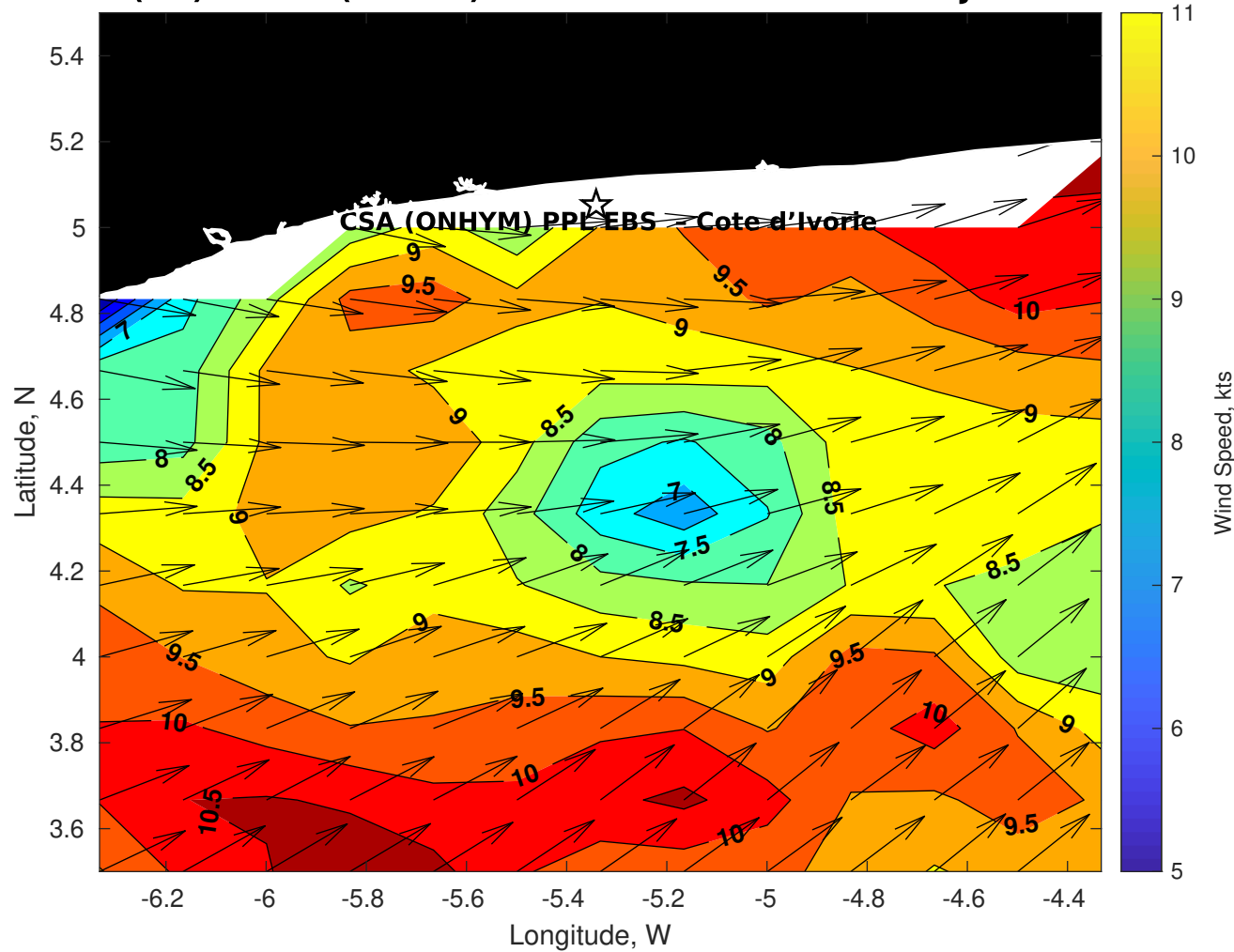
GFS Winds (kts) for CSA (ONHYM) PPL EBS - Cote d'Ivoire at 07-Jan-2026 09:00:00
