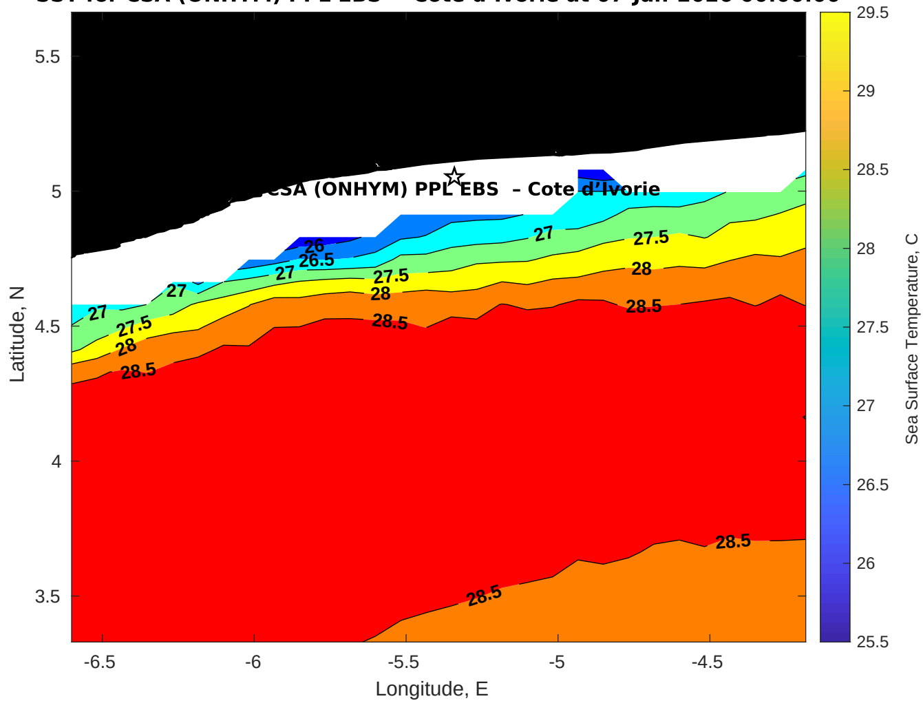
SST for CSA (ONHYM) PPL EBS - Cote d'Ivoire at 07-Jan-2026 00:00:00
