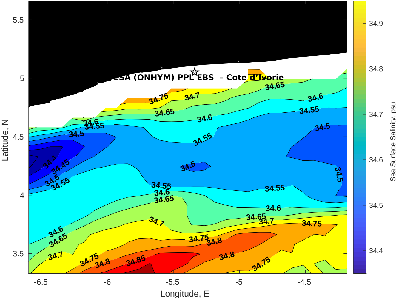
Surface Salinity for CSA (ONHYM) PPL EBS - Cote d'Ivoire at 07-Jan-2026 00:00:00
