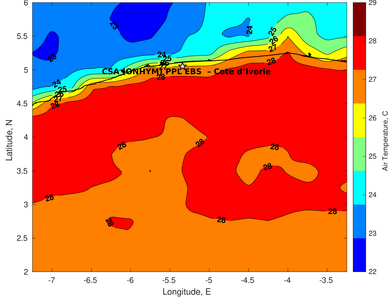
Air Temperature (C) for CSA (ONHYM) PPL EBS - Cote d'Ivoire at 08-Jan-2026
