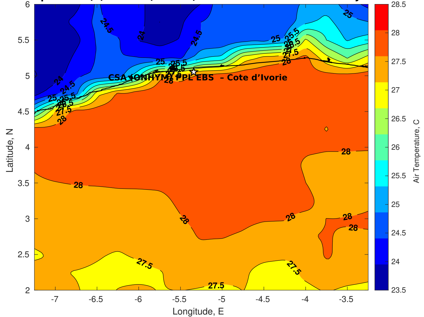
Air Temperature (C) for CSA (ONHYM) PPL EBS - Cote d'Ivoire at 08-Jan-2026
