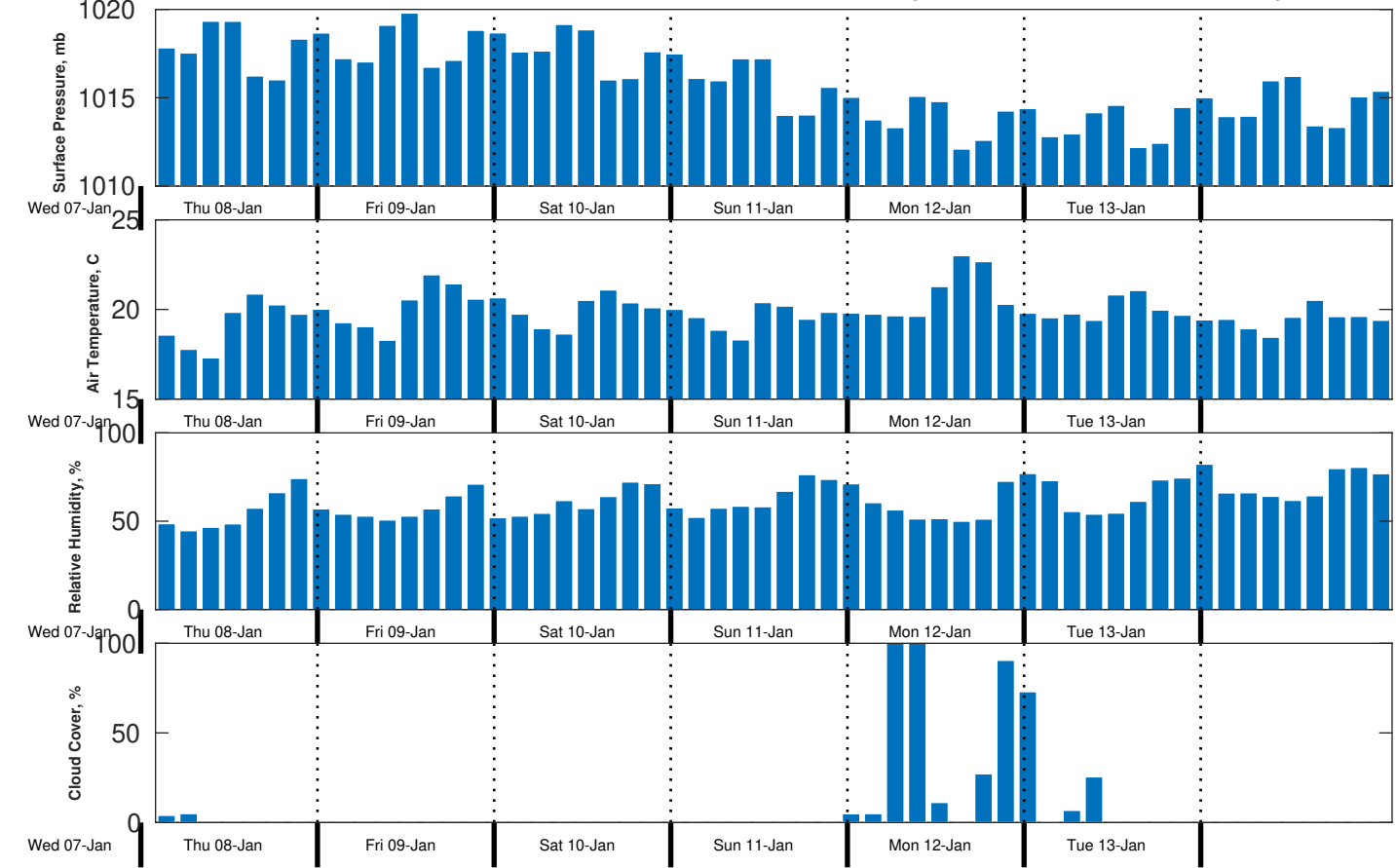
Met Forecast for CSA (ONHYM) PPL EBS - Mauritania from 08-Jan-2026 00:00:00 to 15-Jan-2026 00:00:00
