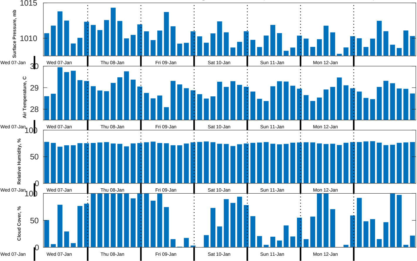
Met Forecast for CSA (ONHYM) PPL EBS - Nigeria from 08-Jan-2026 00:00:00 to 15-Jan-2026 00:00:00
