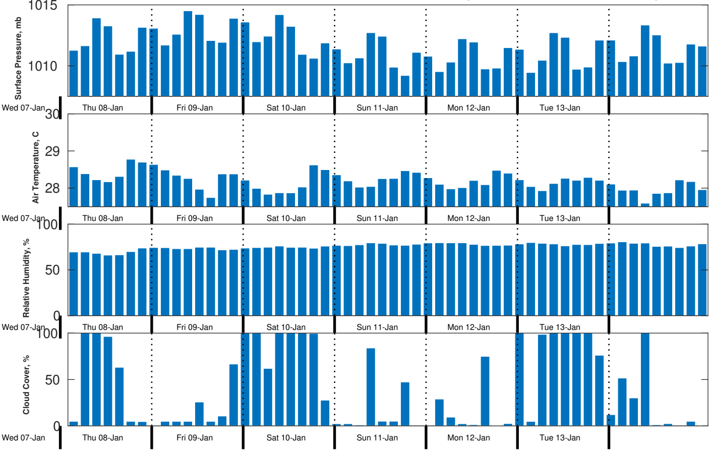
Met Forecast for CSA (ONHYM) PPL EBS - Sierra Leone from 08-Jan-2026 00:00:00 to 15-Jan-2026 00:00:00
