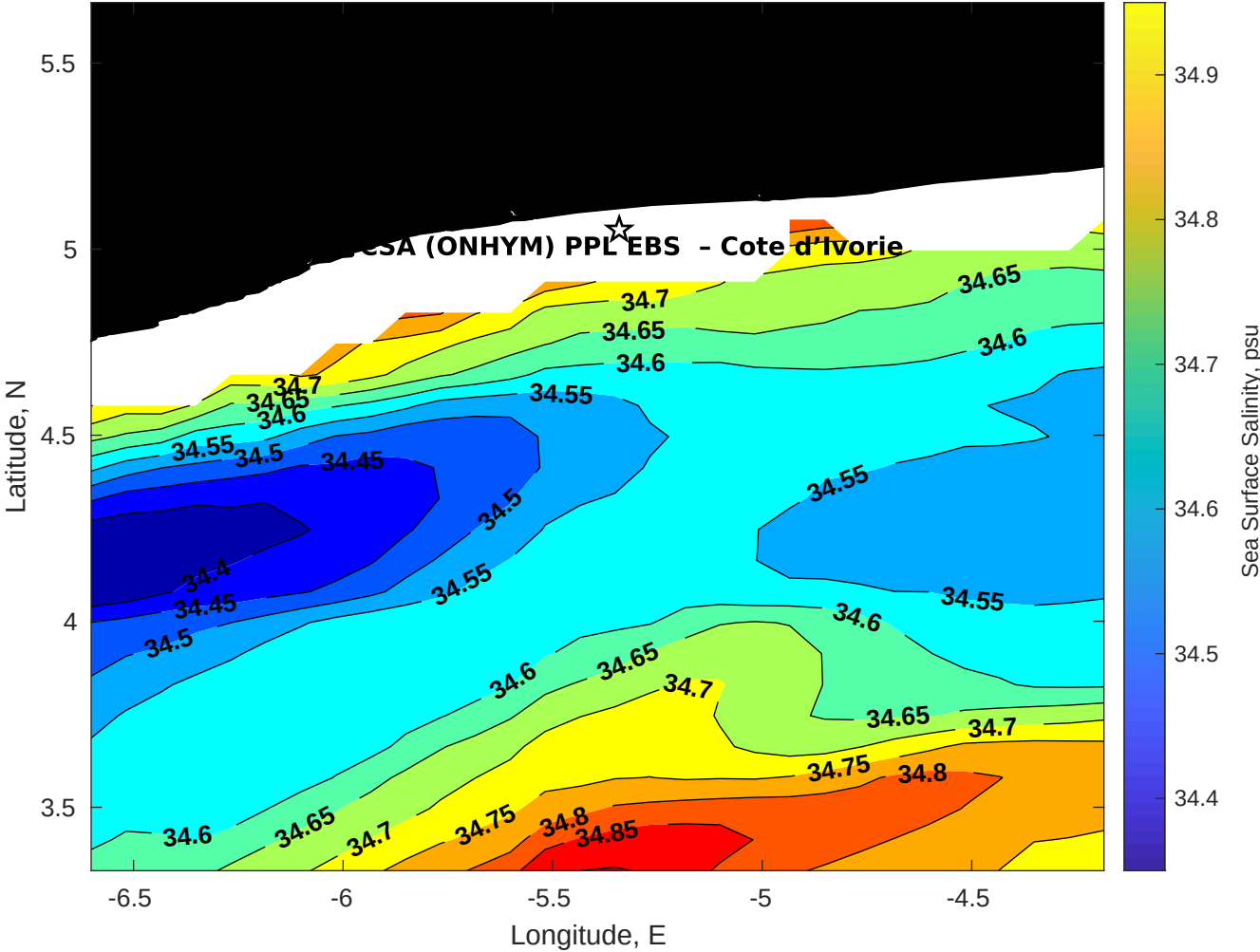
Surface Salinity for CSA (ONHYM) PPL EBS - Cote d'Ivoire at 08-Jan-2026 00:00:00
