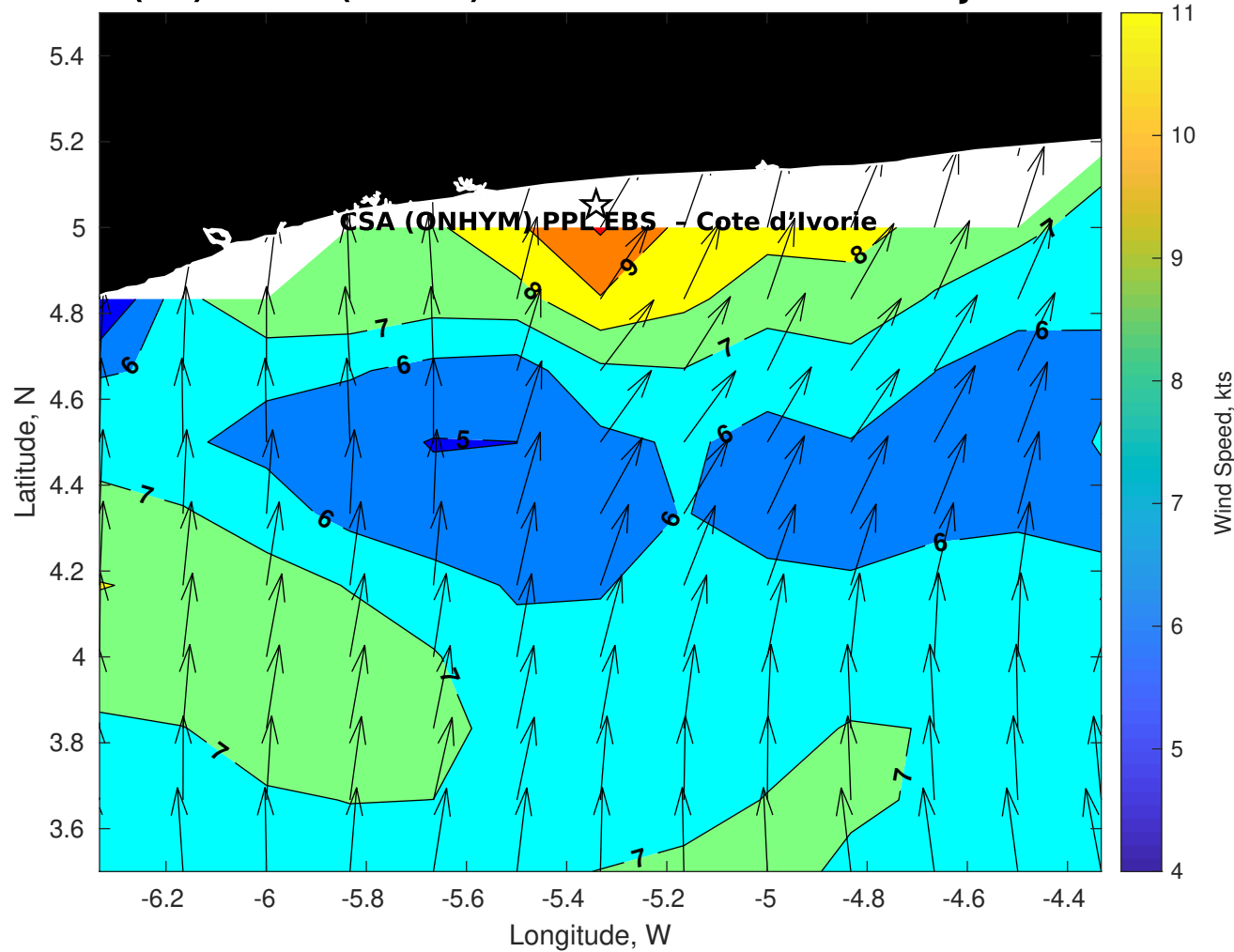
GFS Winds (kts) for CSA (ONHYM) PPL EBS - Cote d'Ivoire at 09-Jan-2026 09:00:00
