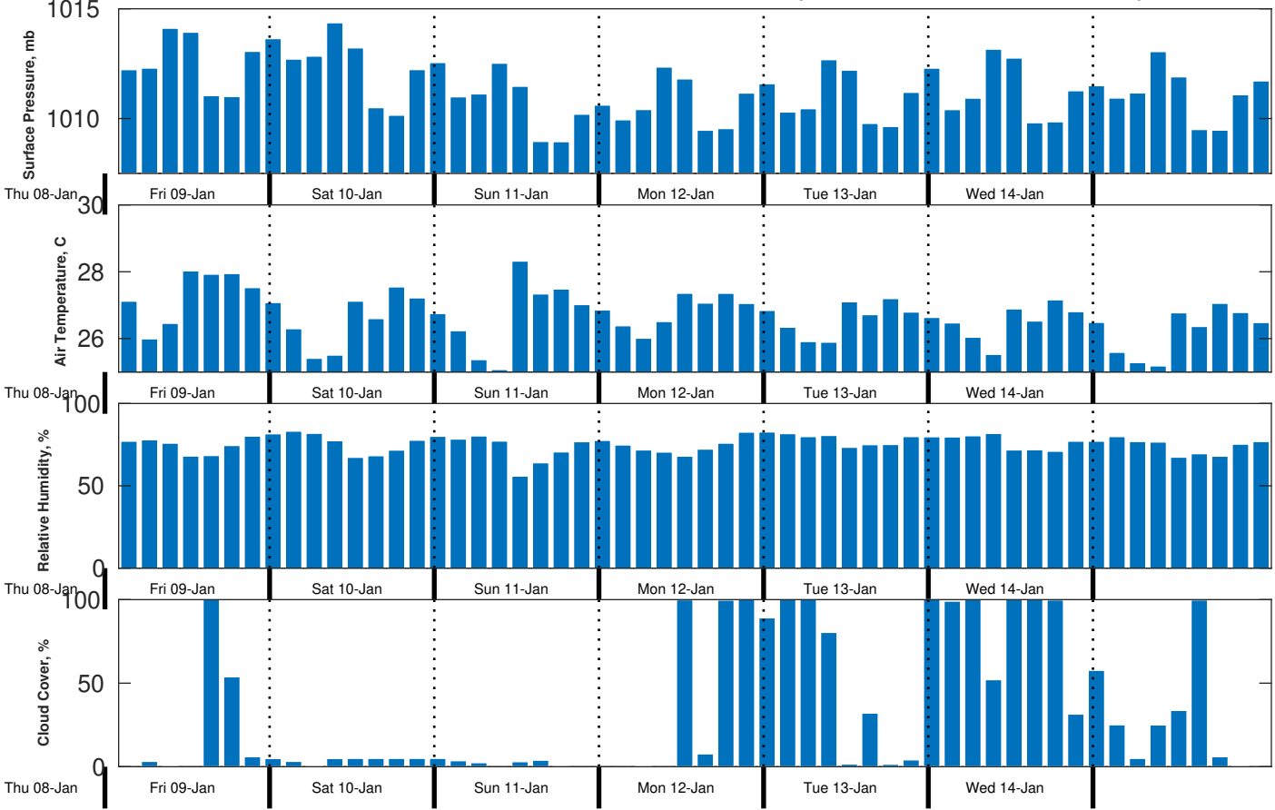
Met Forecast for CSA (ONHYM) PPL EBS - Guinea from 09-Jan-2026 00:00:00 to 16-Jan-2026 00:00:00
