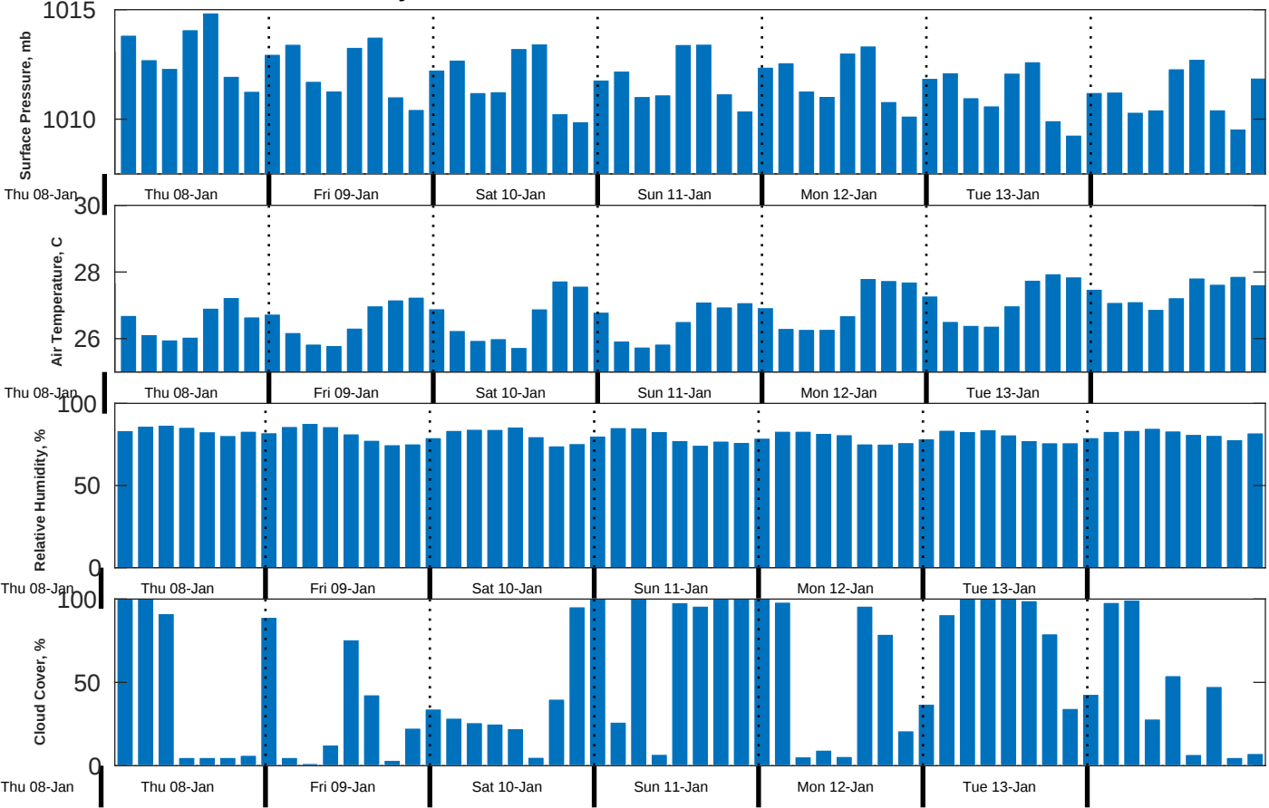
Met Forecast for Gyre from 08-Jan-2026 20:00:00 to 15-Jan-2026 20:00:00
