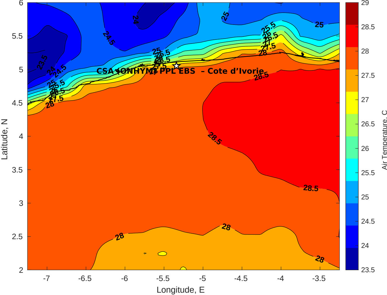
Air Temperature (C) for CSA (ONHYM) PPL EBS - Cote d'Ivoire at 10-Jan-2026
