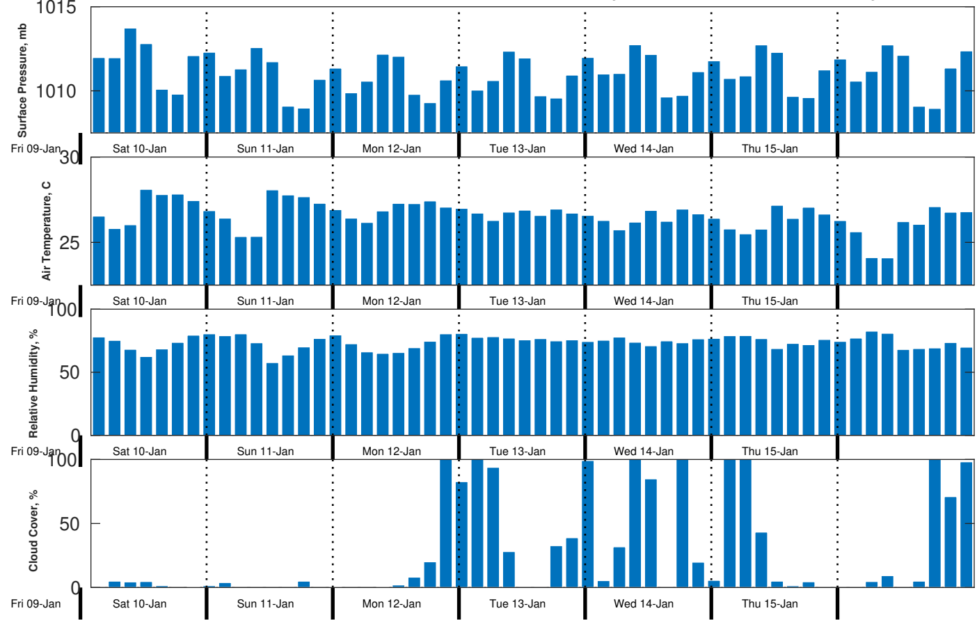
Met Forecast for CSA (ONHYM) PPL EBS - Guinea from 10-Jan-2026 00:00:00 to 17-Jan-2026 00:00:00
