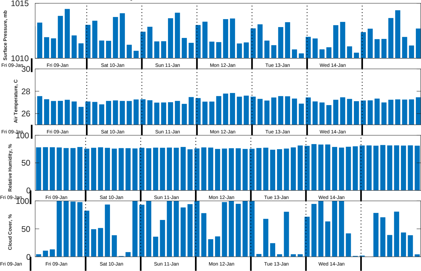
Met Forecast for Gyre from 09-Jan-2026 20:00:00 to 16-Jan-2026 20:00:00
