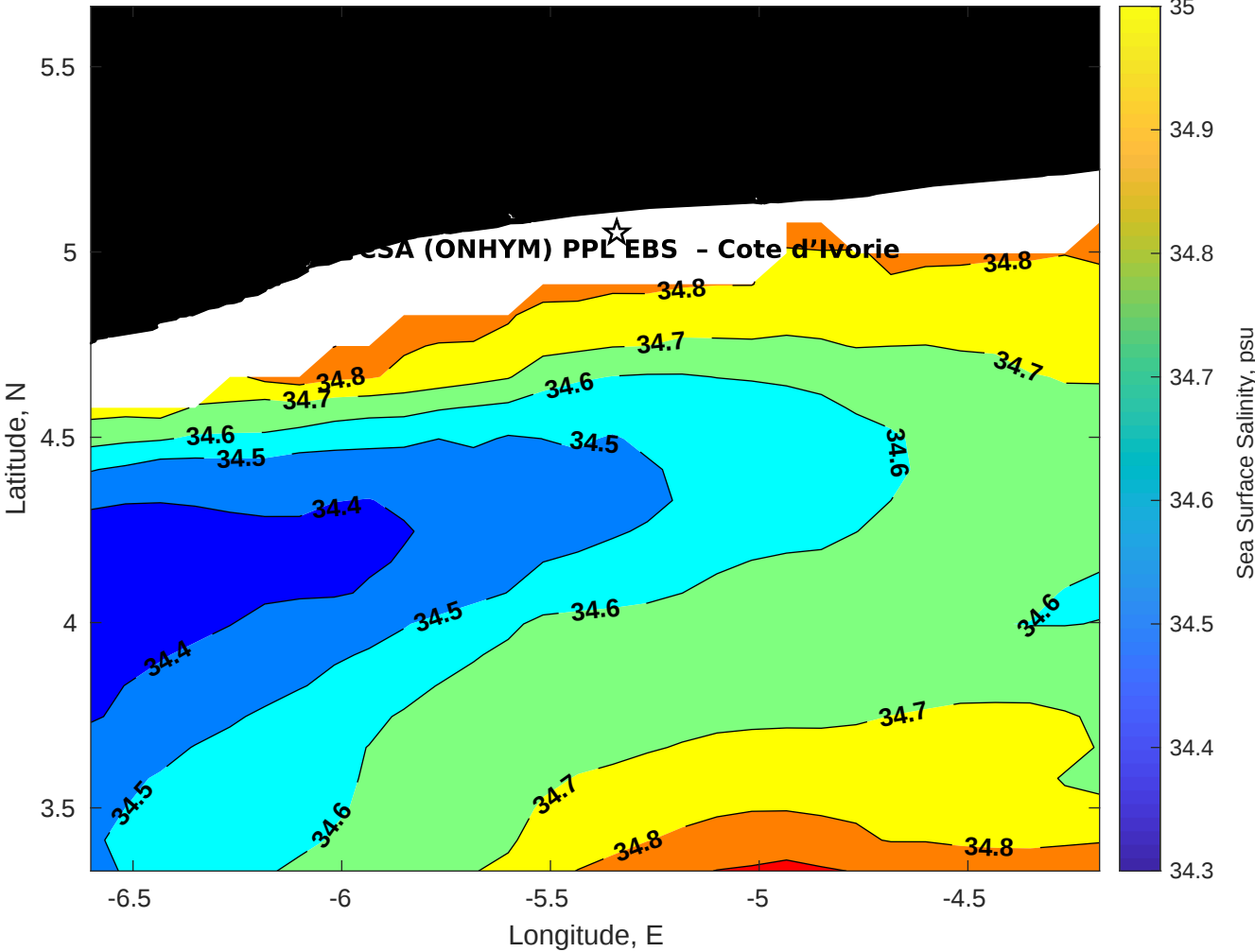
Surface Salinity for CSA (ONHYM) PPL EBS - Cote d'Ivoire at 10-Jan-2026 00:00:00
