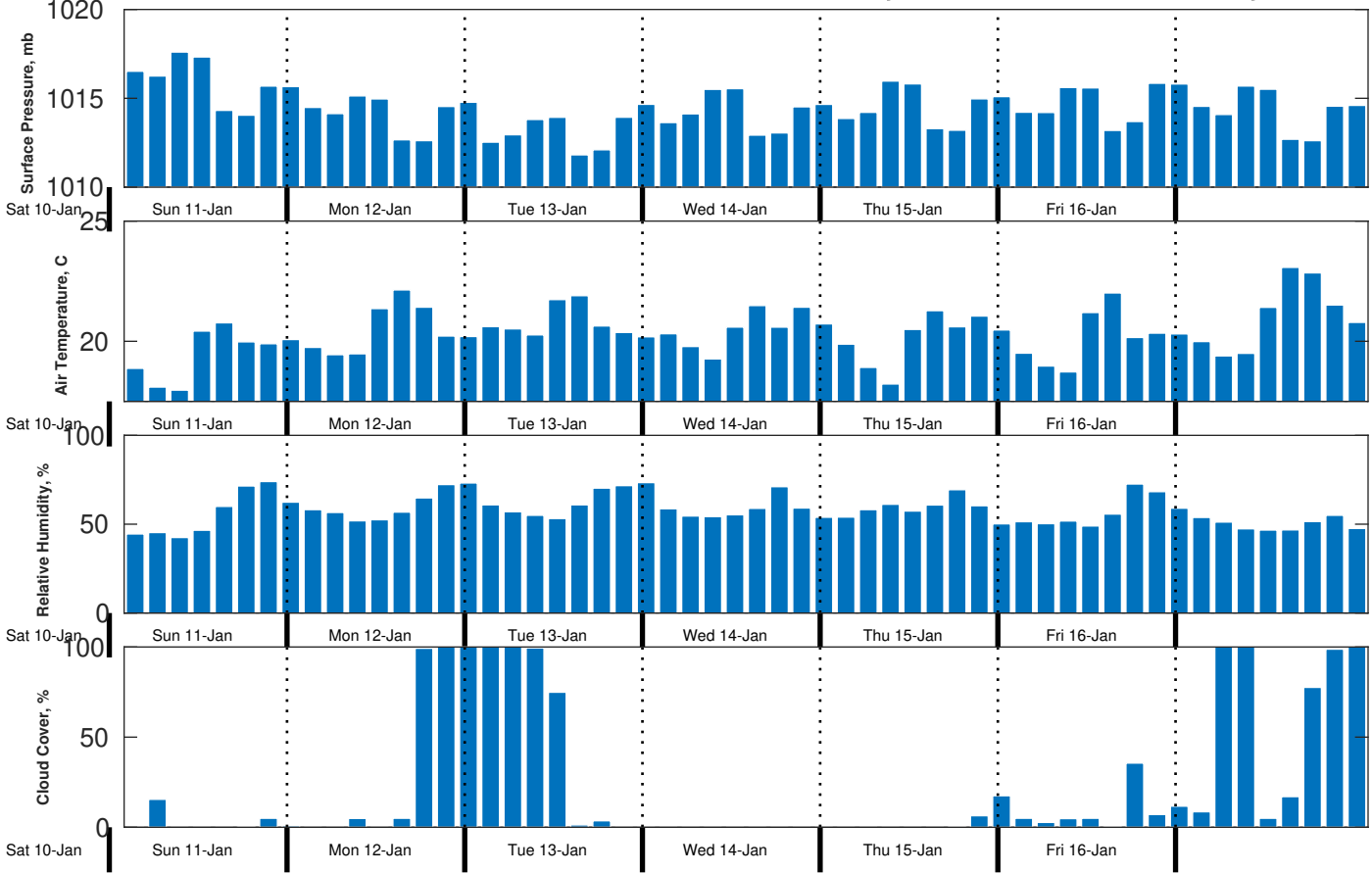
Met Forecast for CSA (ONHYM) PPL EBS - Mauritania from 11-Jan-2026 00:00:00 to 18-Jan-2026 00:00:00
