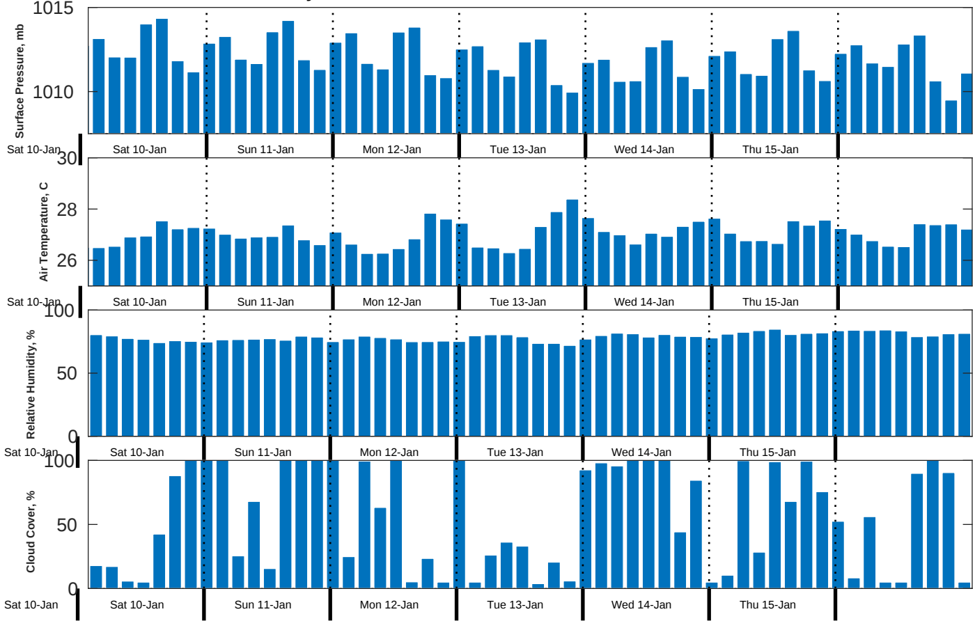
Met Forecast for Gyre from 10-Jan-2026 20:00:00 to 17-Jan-2026 20:00:00
