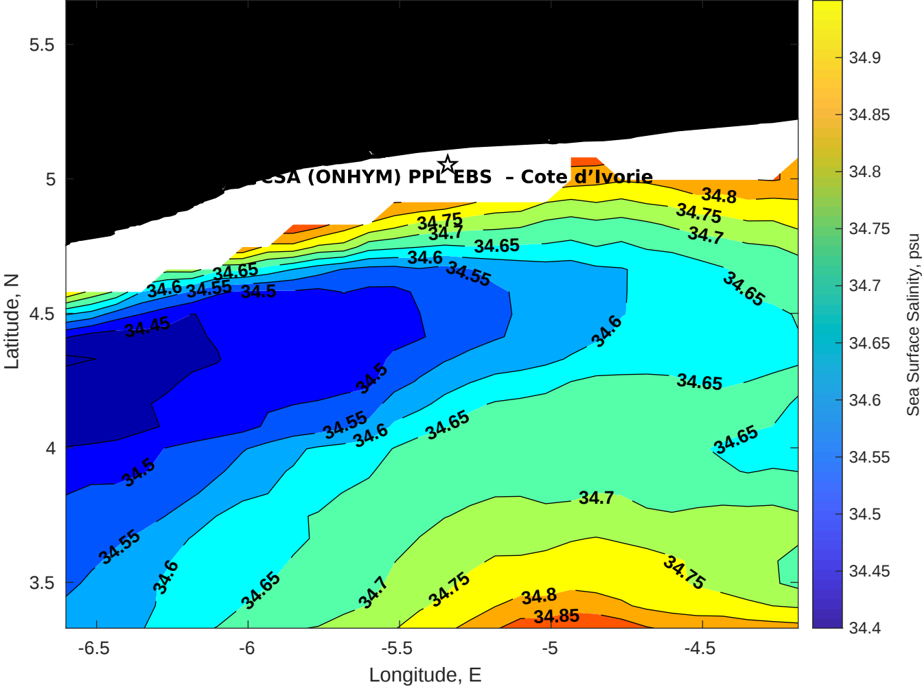
Surface Salinity for CSA (ONHYM) PPL EBS - Cote d'Ivoire at 11-Jan-2026 00:00:00
