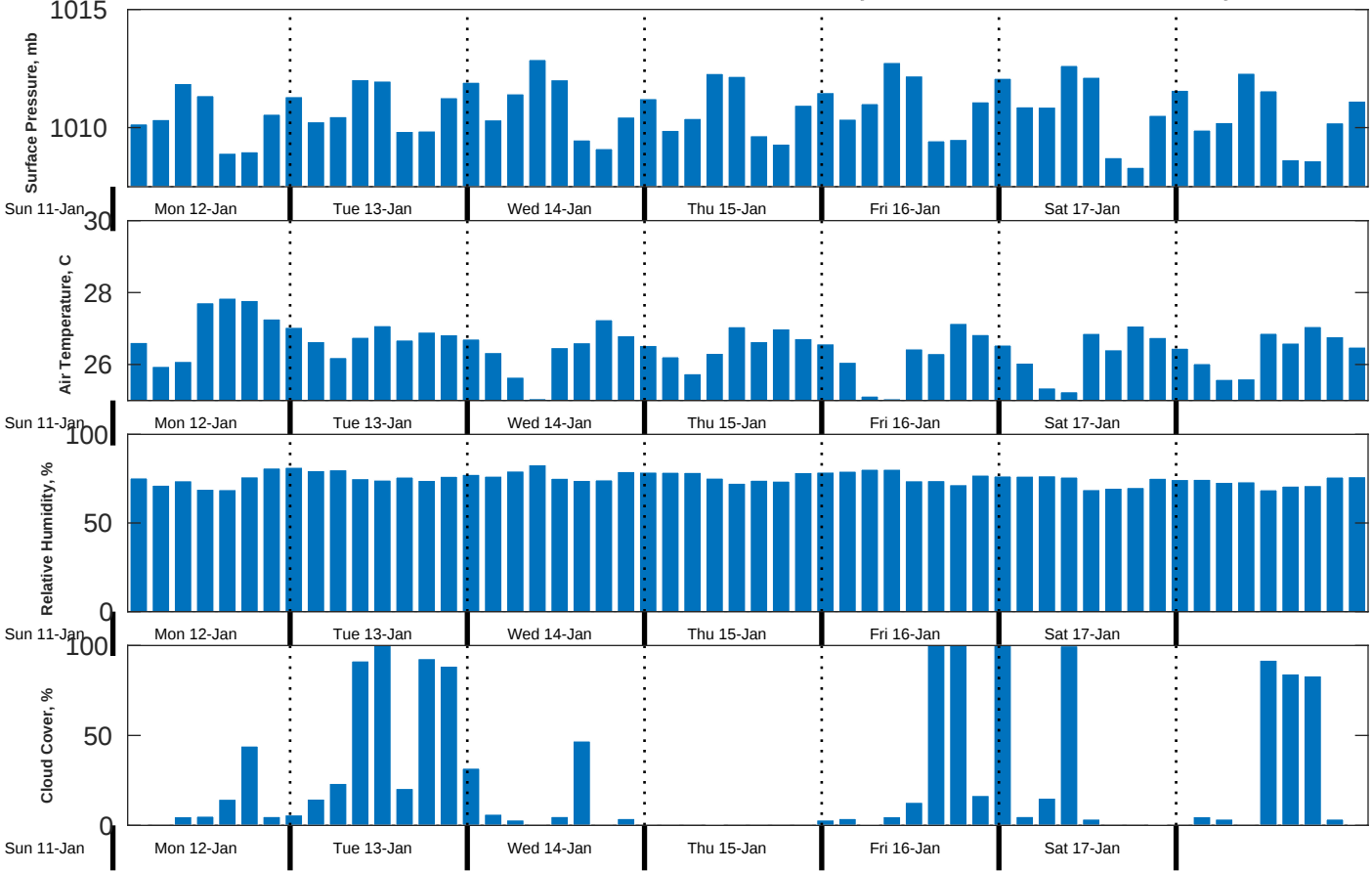
Met Forecast for CSA (ONHYM) PPL EBS - Guinea from 12-Jan-2026 00:00:00 to 19-Jan-2026 00:00:00
