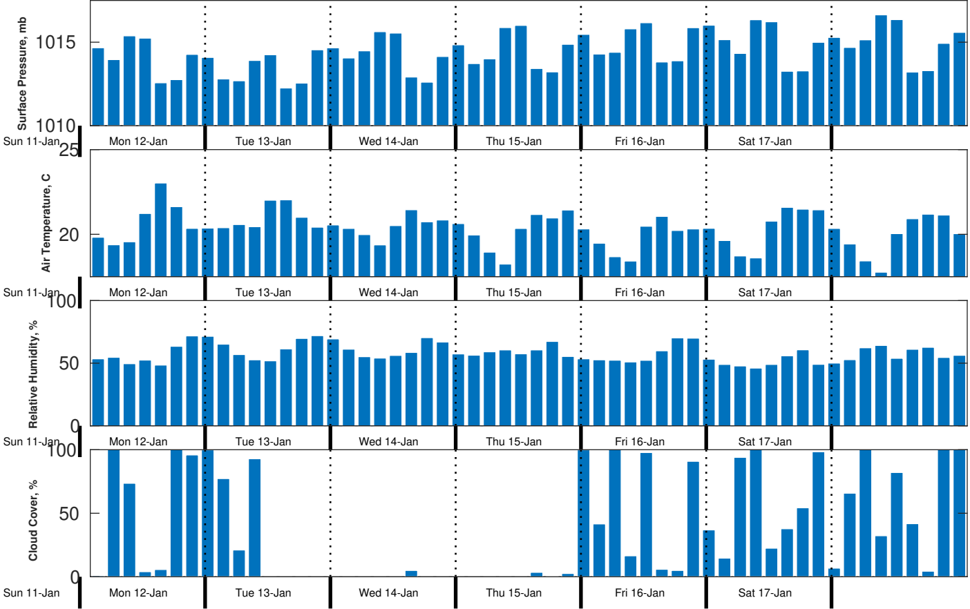
Met Forecast for CSA (ONHYM) PPL EBS - Mauritania from 12-Jan-2026 00:00:00 to 19-Jan-2026 00:00:00
