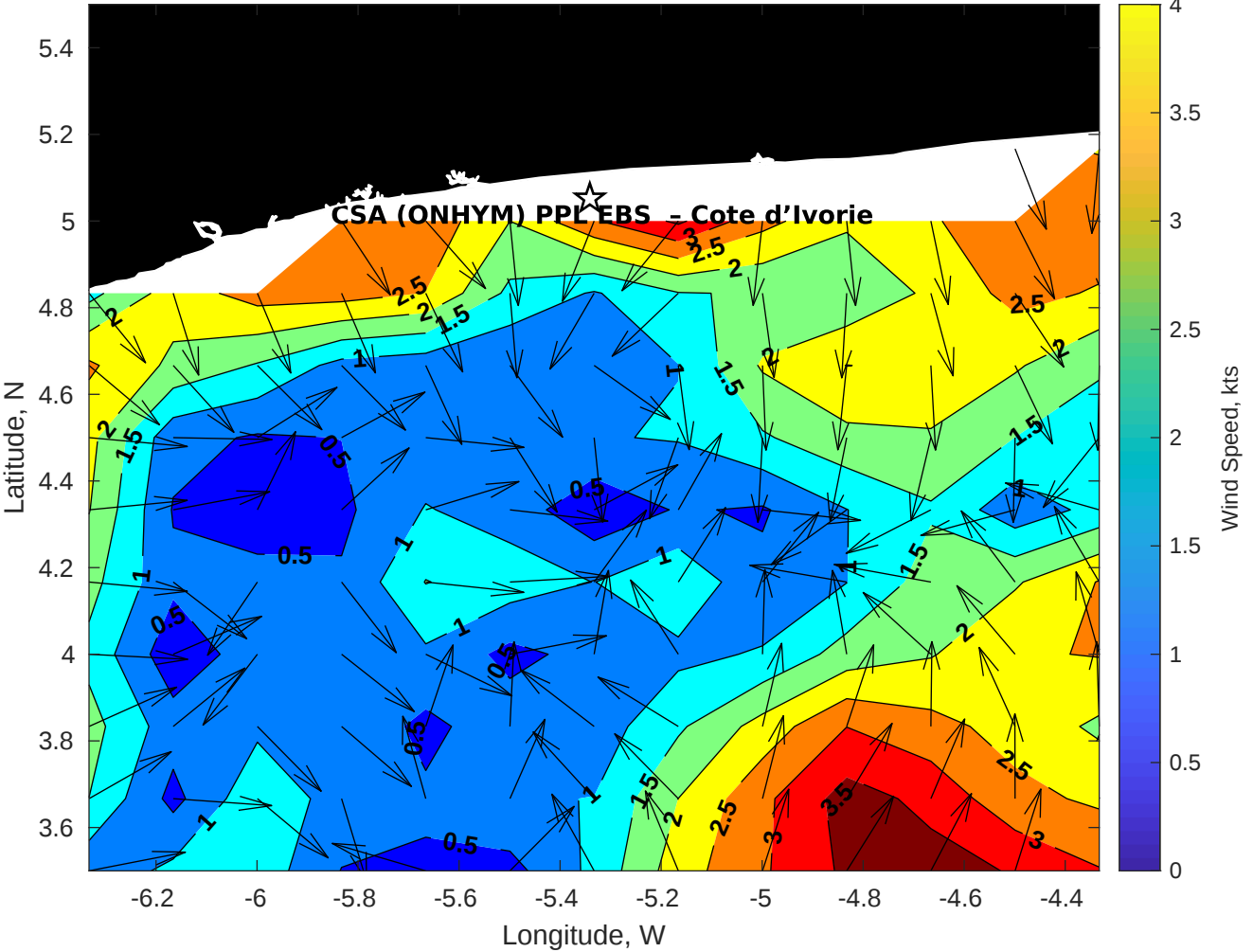
GFS Winds (kts) for CSA (ONHYM) PPL EBS - Cote d'Ivoire at 13-Jan-2026 09:00:00
