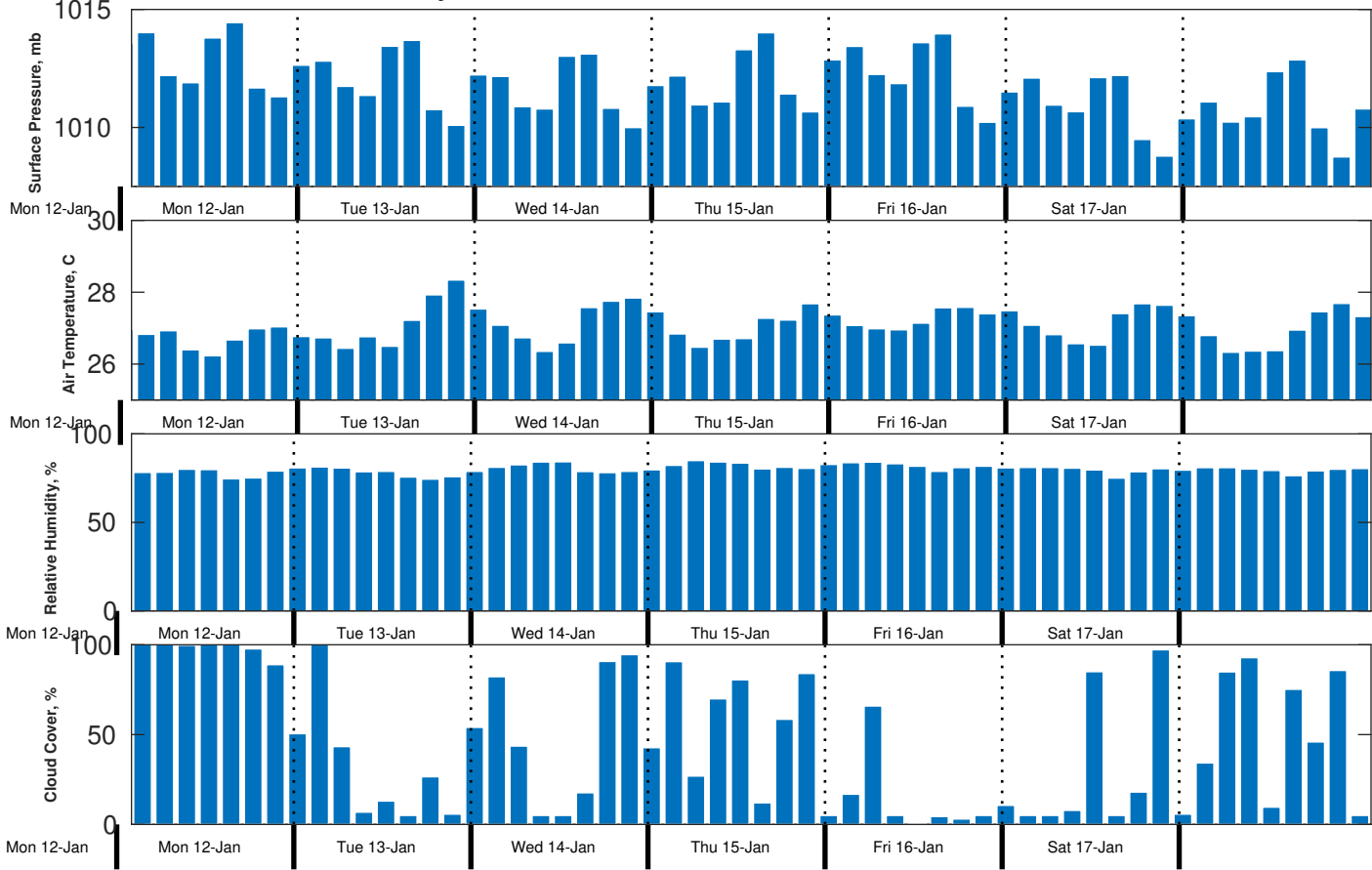
Met Forecast for Gyre from 12-Jan-2026 20:00:00 to 19-Jan-2026 20:00:00
