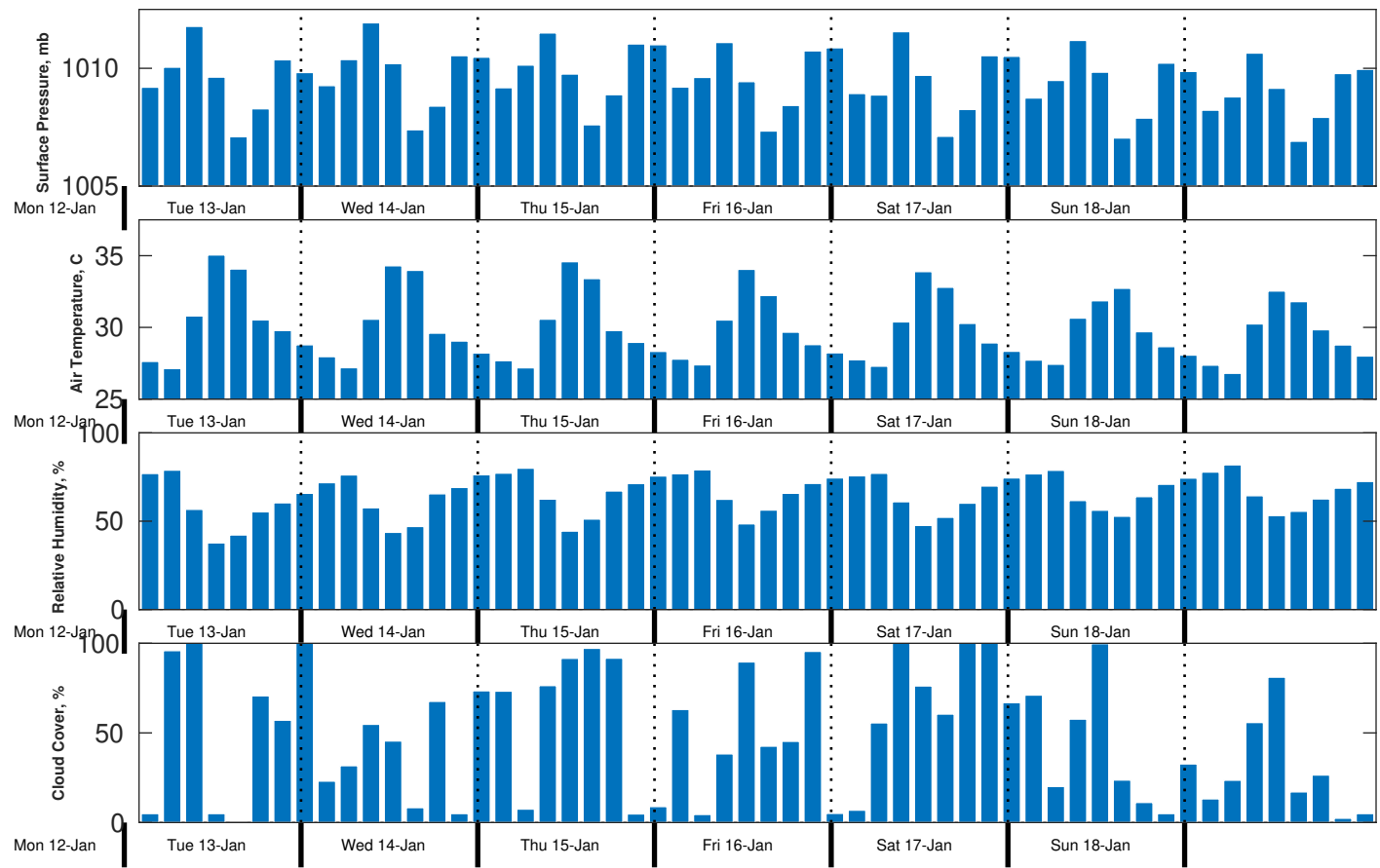
Met Forecast for Proteus from 13-Jan-2026 00:00:00 to 20-Jan-2026 00:00:00
