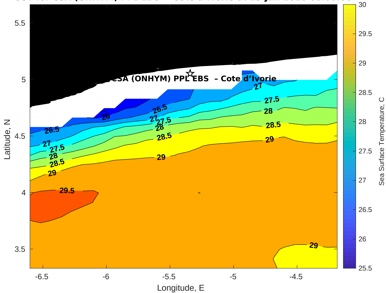
SST for CSA (ONHYM) PPL EBS - Cote d'Ivoire at 13-Jan-2026 00:00:00
