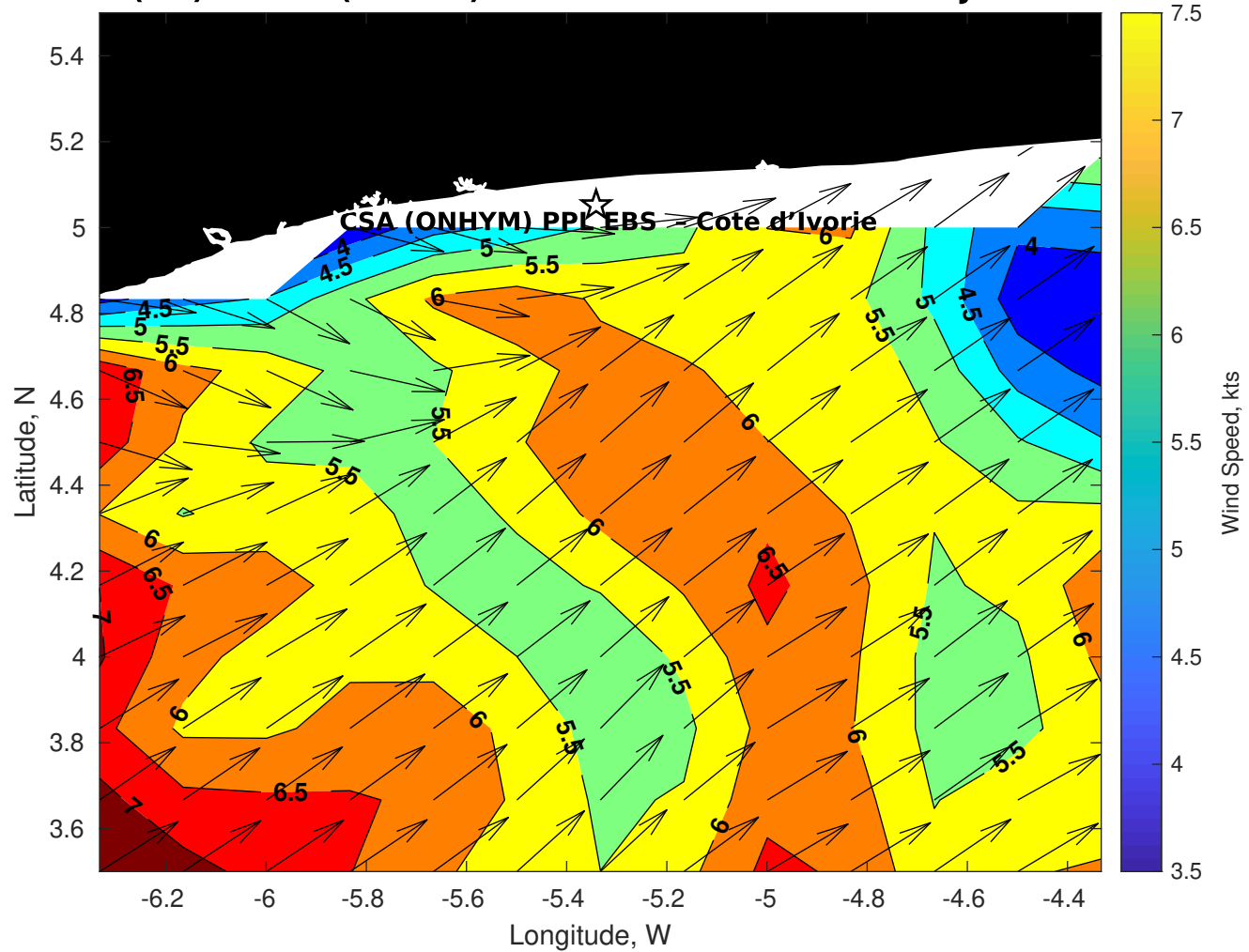
GFS Winds (kts) for CSA (ONHYM) PPL EBS - Cote d'Ivoire at 14-Jan-2026 09:00:00
