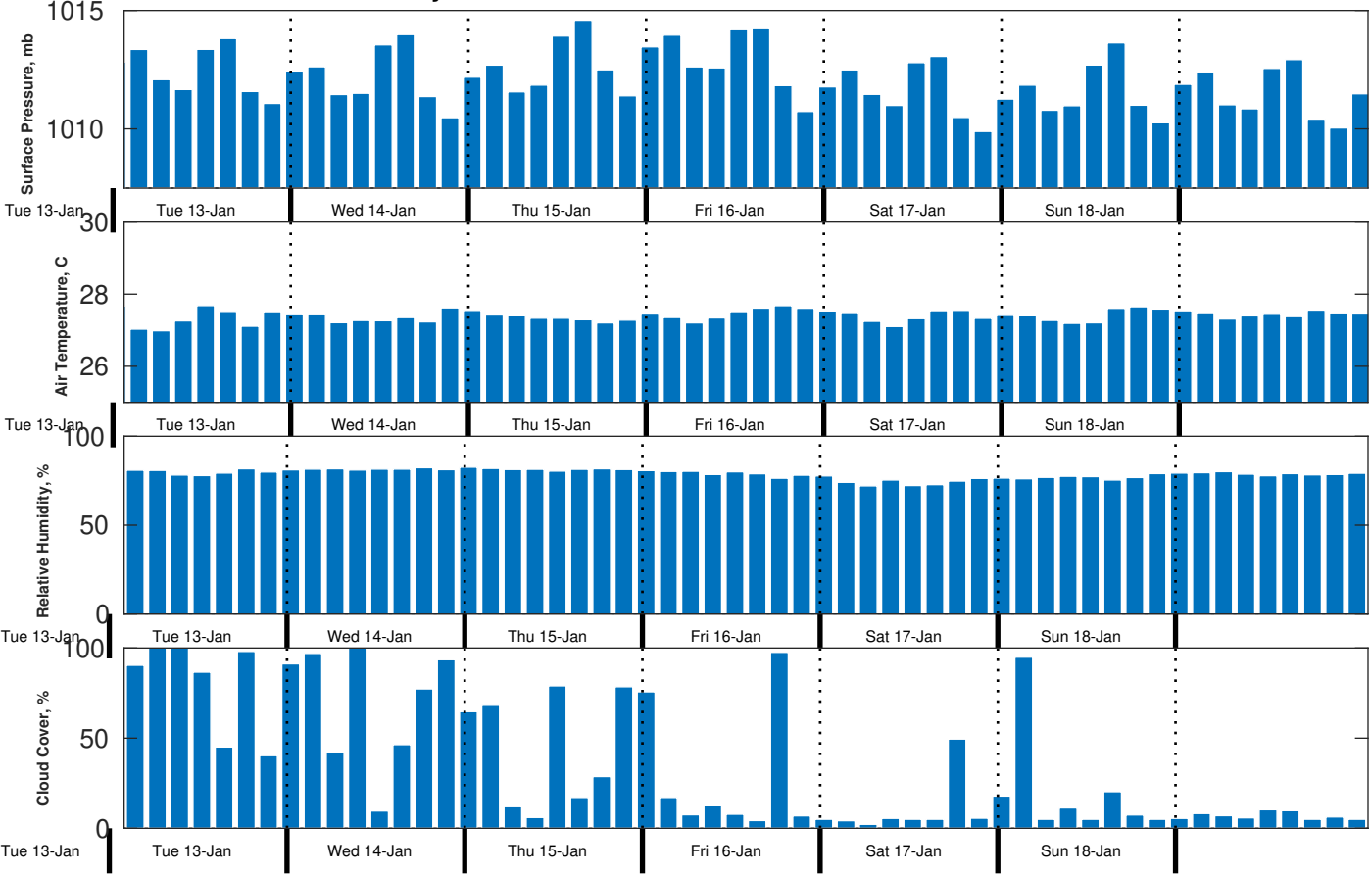
Met Forecast for Gyre from 13-Jan-2026 20:00:00 to 20-Jan-2026 20:00:00
