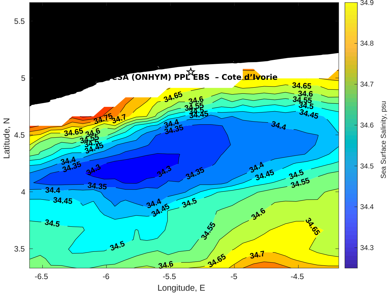
Surface Salinity for CSA (ONHYM) PPL EBS - Cote d'Ivoire at 14-Jan-2026 00:00:00
