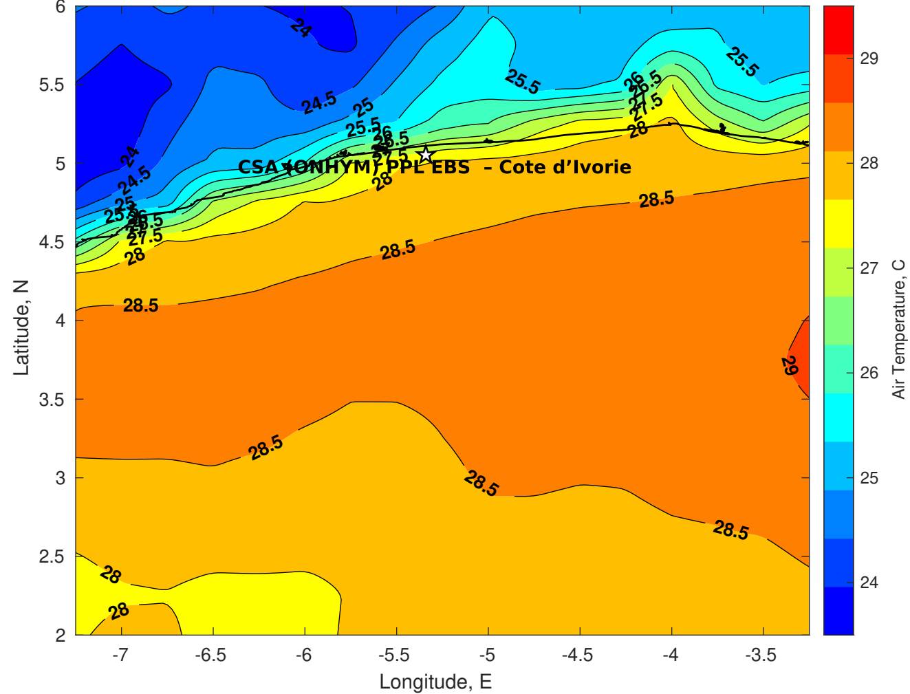
Air Temperature (C) for CSA (ONHYM) PPL EBS - Cote d'Ivoire at 15-Jan-2026
