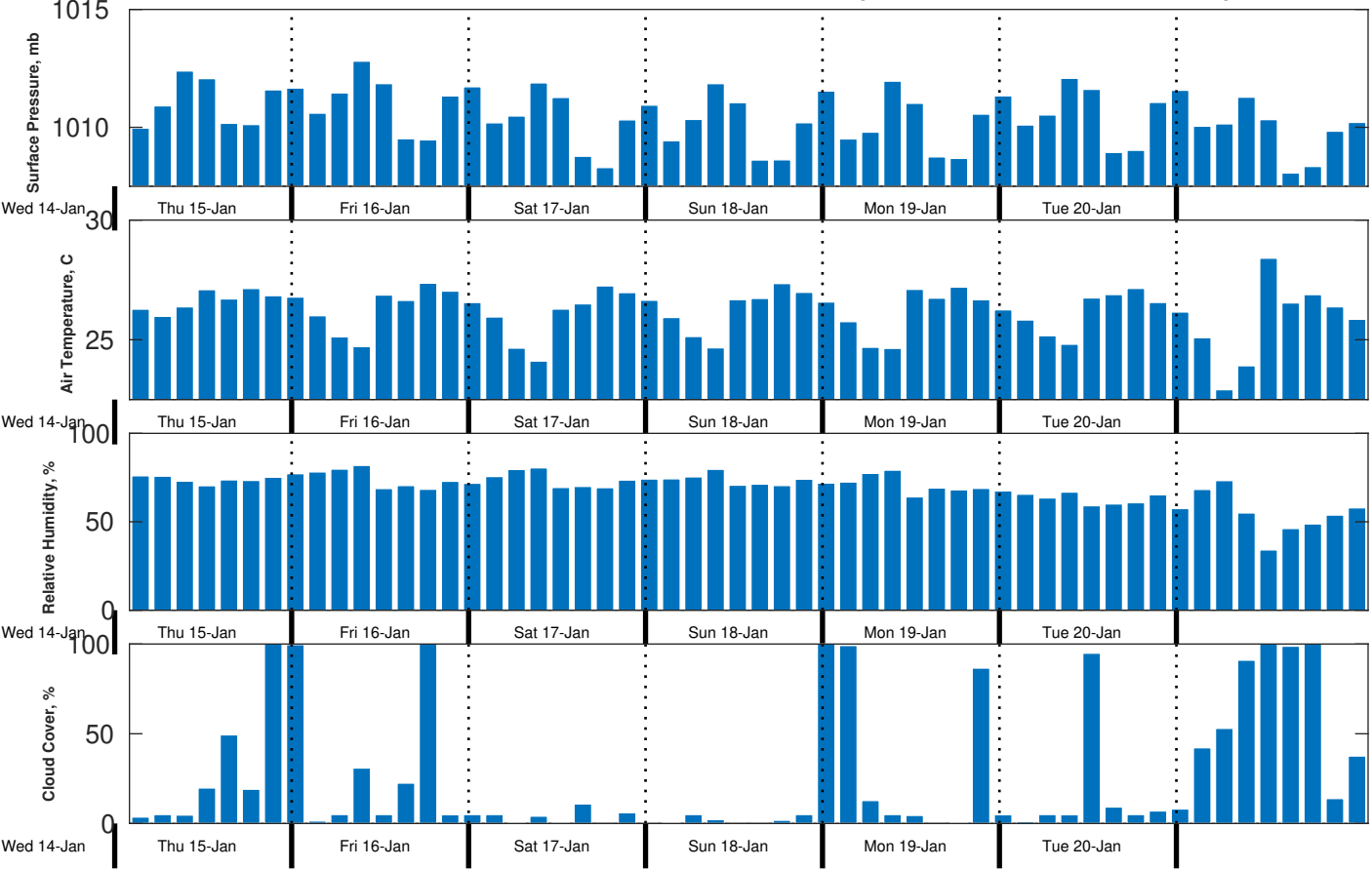
Met Forecast for CSA (ONHYM) PPL EBS - Guinea from 15-Jan-2026 00:00:00 to 22-Jan-2026 00:00:00
