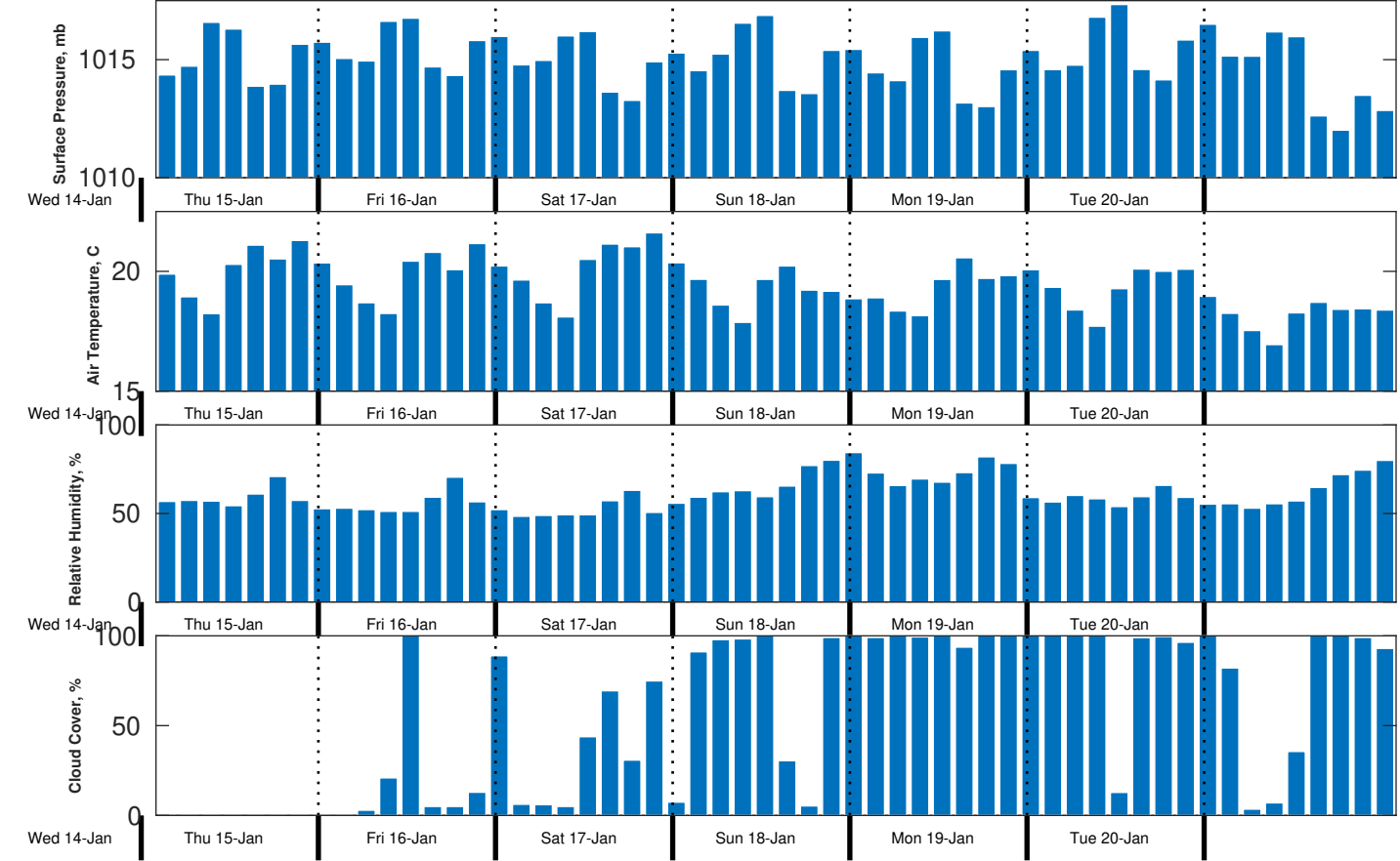
Met Forecast for CSA (ONHYM) PPL EBS - Mauritania from 15-Jan-2026 00:00:00 to 22-Jan-2026 00:00:00
