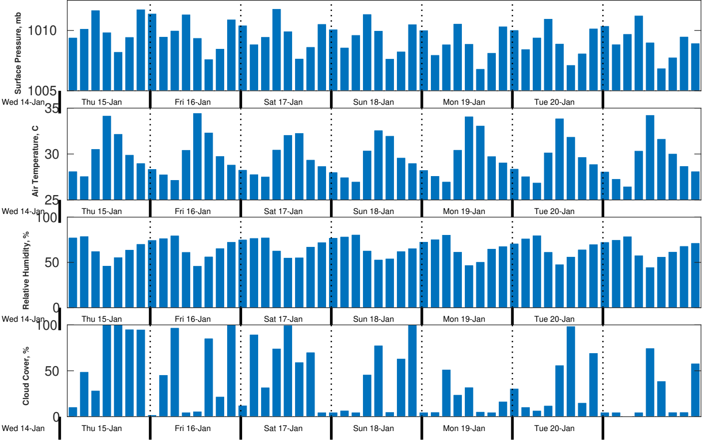
Met Forecast for Proteus from 15-Jan-2026 00:00:00 to 22-Jan-2026 00:00:00
