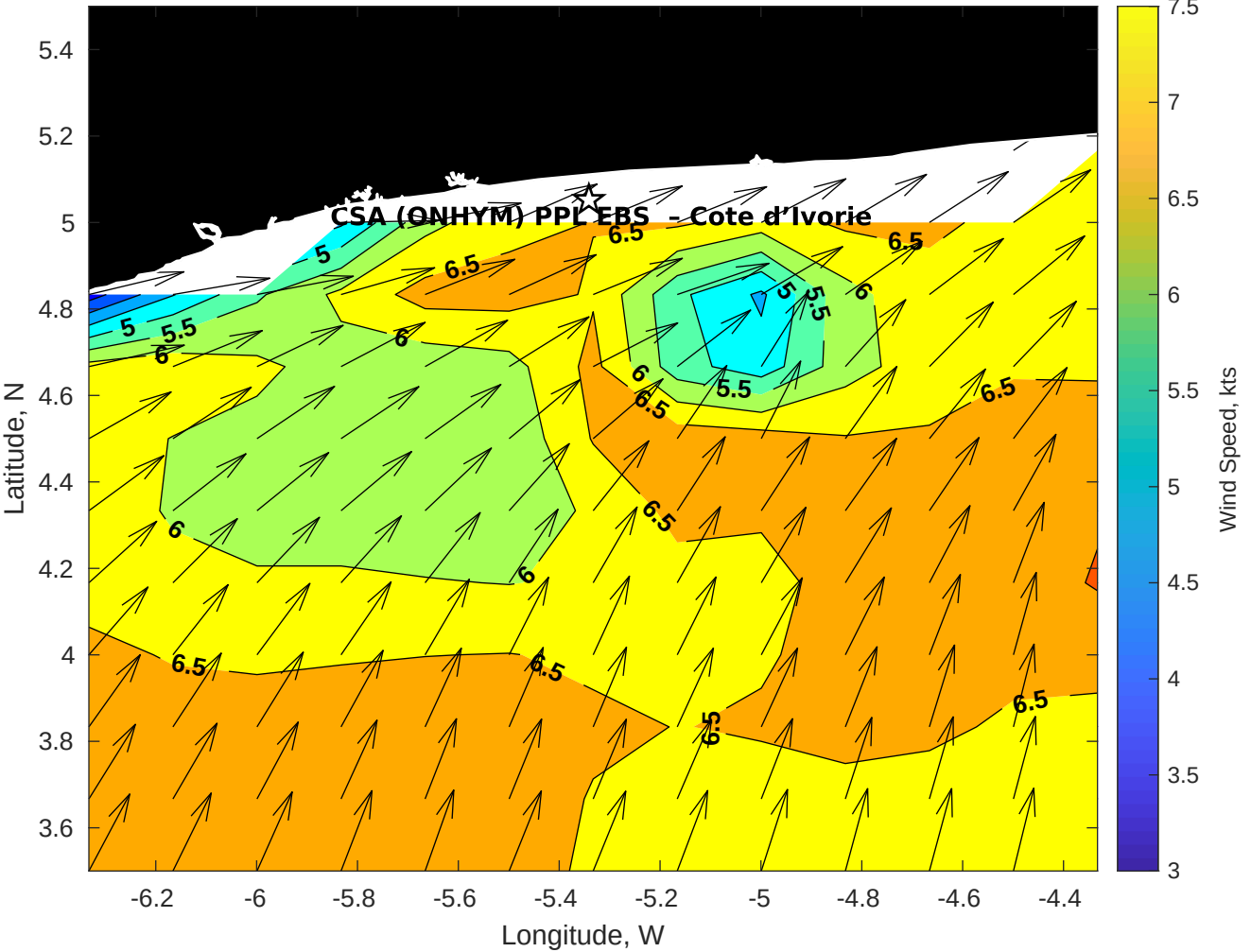
GFS Winds (kts) for CSA (ONHYM) PPL EBS - Cote d'Ivoire at 16-Jan-2026 09:00:00
