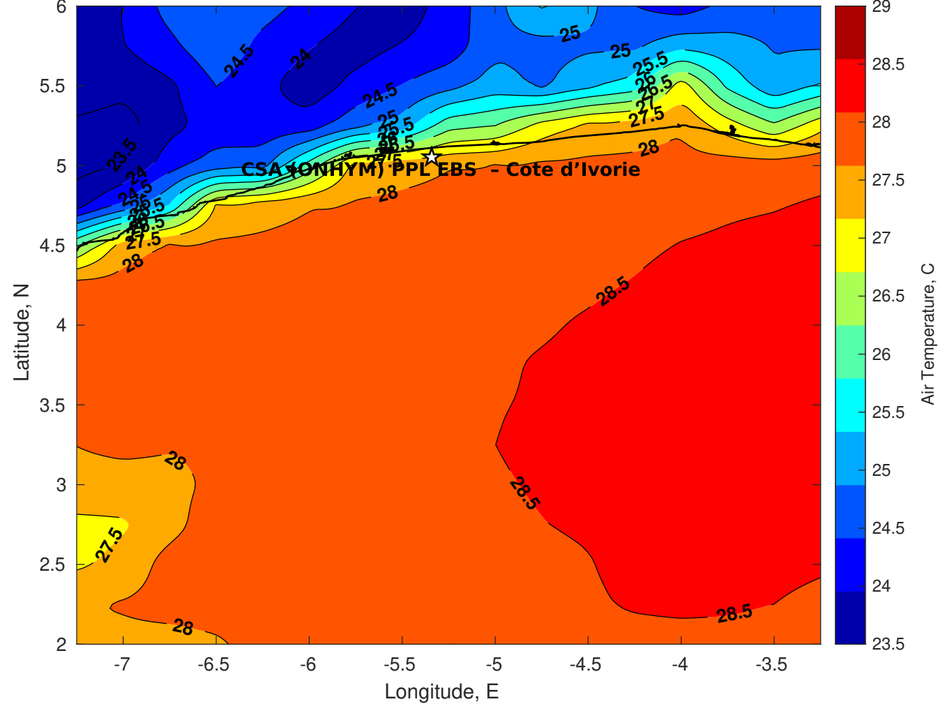
Air Temperature (C) for CSA (ONHYM) PPL EBS - Cote d'Ivoire at 16-Jan-2026
