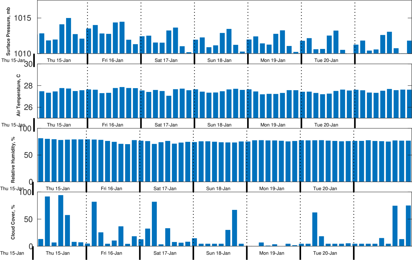
Met Forecast for Gyre from 15-Jan-2026 20:00:00 to 22-Jan-2026 20:00:00
