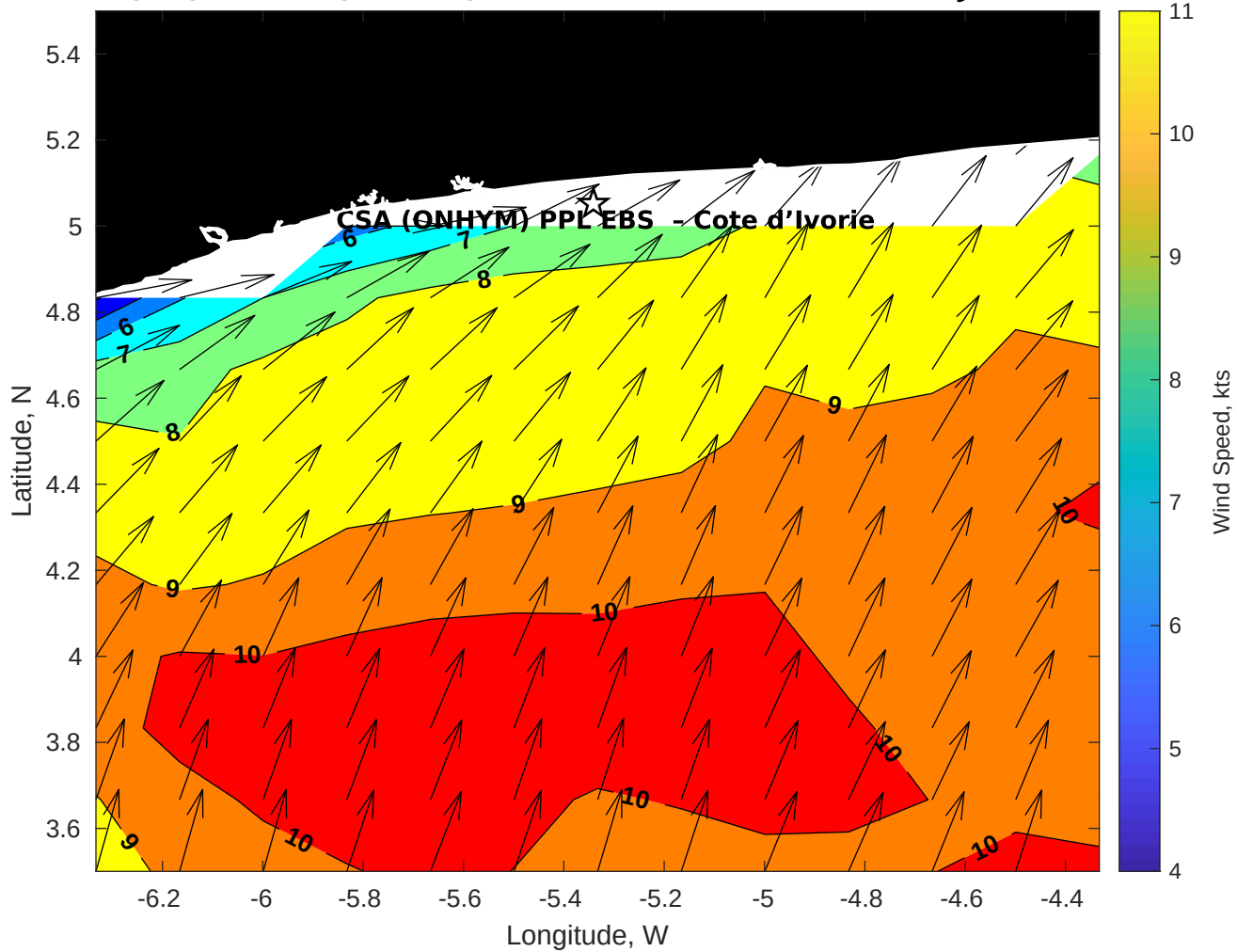
GFS Winds (kts) for CSA (ONHYM) PPL EBS - Cote d'Ivoire at 18-Jan-2026 09:00:00
