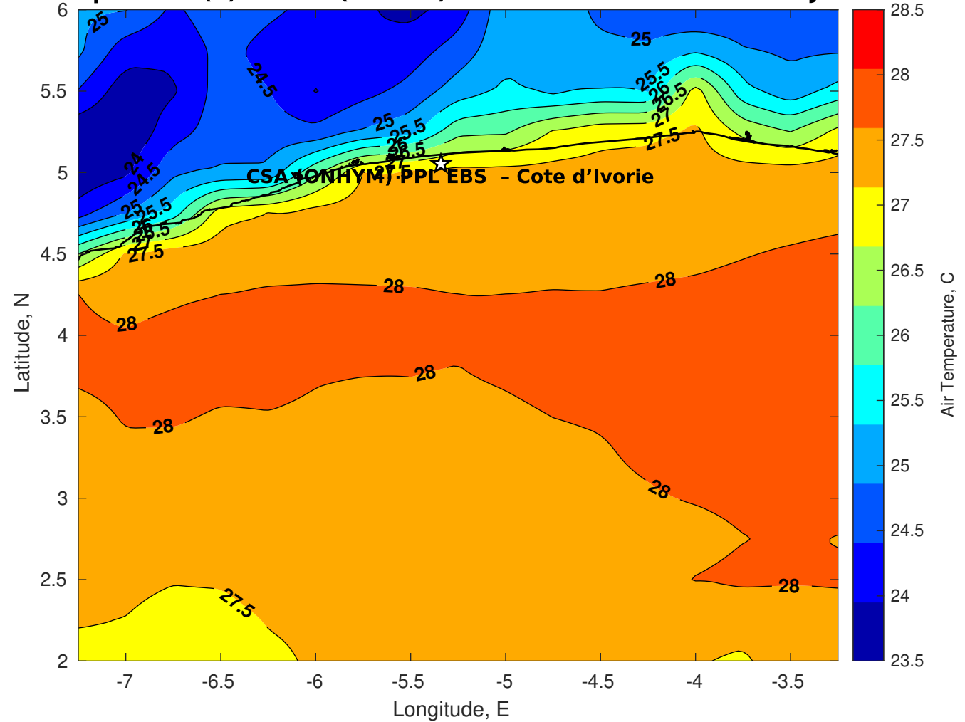
Air Temperature (C) for CSA (ONHYM) PPL EBS - Cote d'Ivoire at 18-Jan-2026
