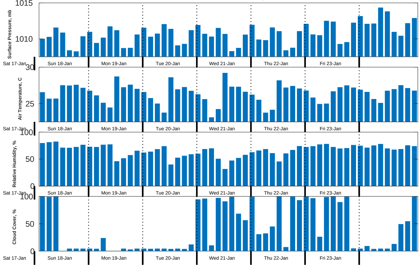
Met Forecast for CSA (ONHYM) PPL EBS - Guinea from 18-Jan-2026 00:00:00 to 25-Jan-2026 00:00:00
