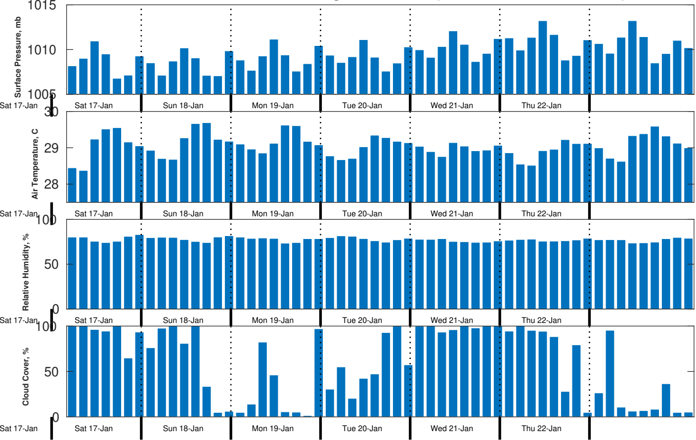
Met Forecast for CSA (ONHYM) PPL EBS - Nigeria from 18-Jan-2026 00:00:00 to 25-Jan-2026 00:00:00
